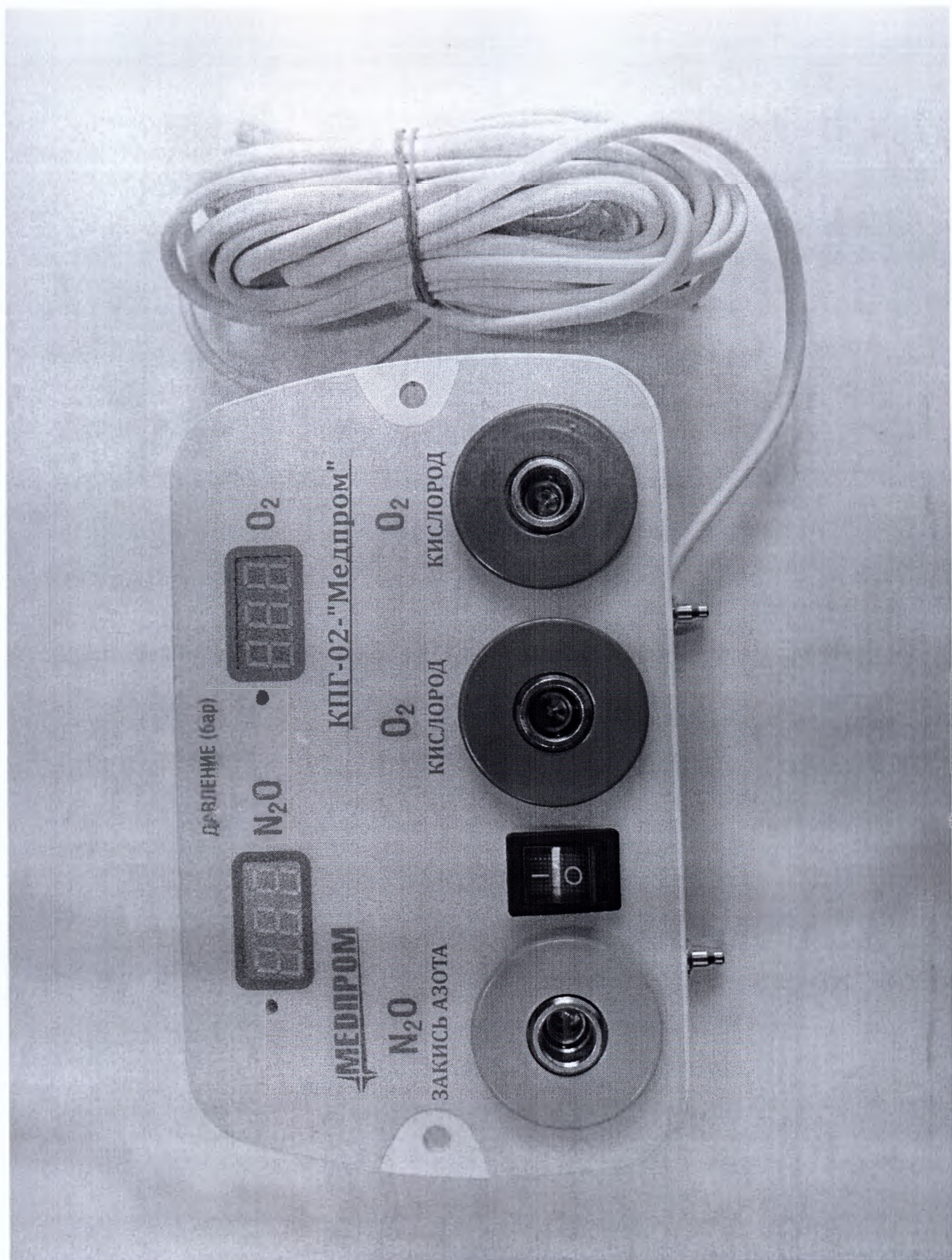
Фотография 2. Комплекс подачи медицинских газов КПГ-«Медпром» по ТУ 9452-006-50063260-2010, исполнение 2: КПГ-02-«Медпром». Общий вид.
