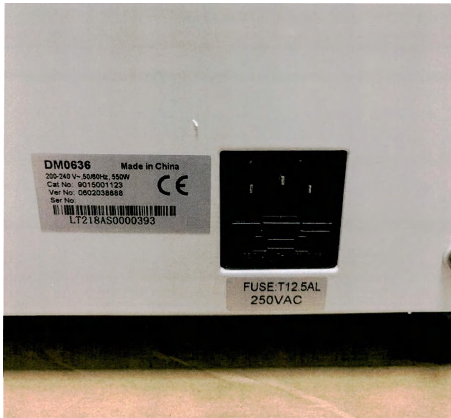
Маркировка центрифуги
