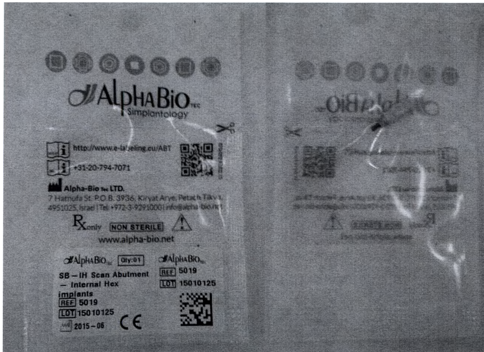
Абатмент сканируемый для стандартной платформы: 5019 SB-IH
