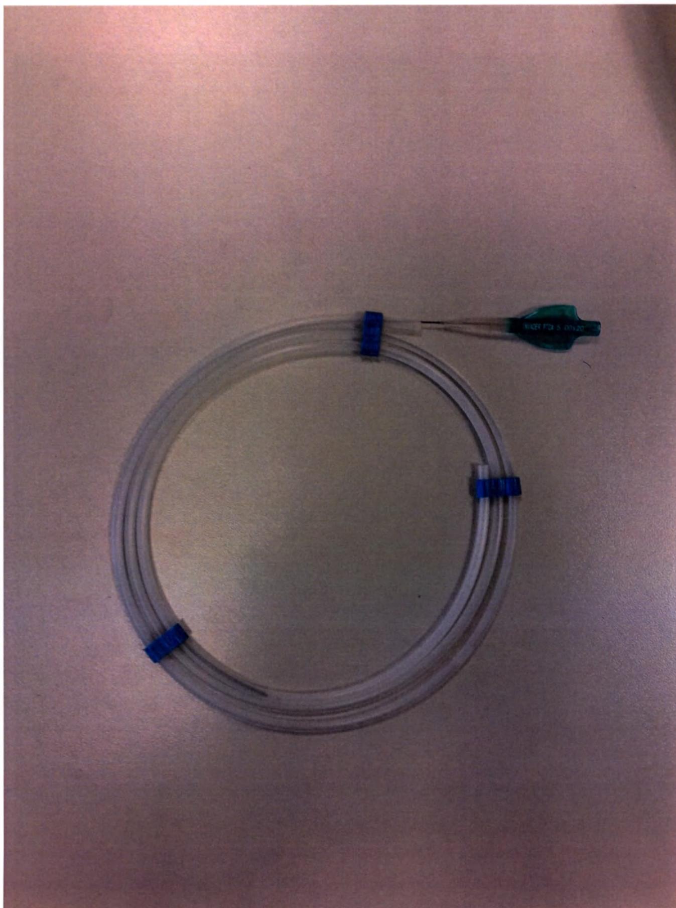
Фото 2. Внешний вид катетера в защитной трубке. Внешний вид катетеров в защитной трубке, зафиксированной клипсами, с различными размерами баллонов идентичен приведенному.
