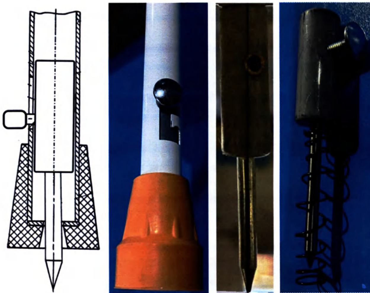
Рис А.7 Устройство противоскольжения (УПС) medshi® М-001 (для вариантов исполнения Костыль подмышечный medshi® Y-01.1, Костыль локтевой medshi® Y-02.1)
