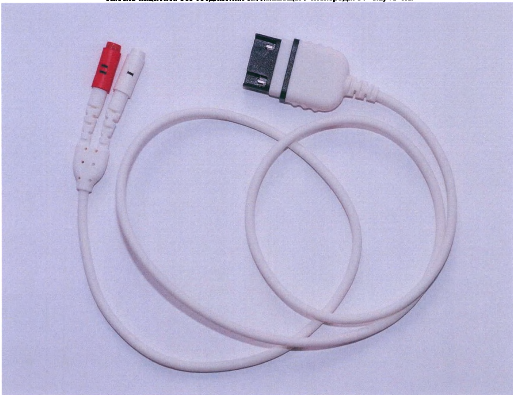
Кабель пациента без соединения заземляющего электрода: 37 см; 75 см.
