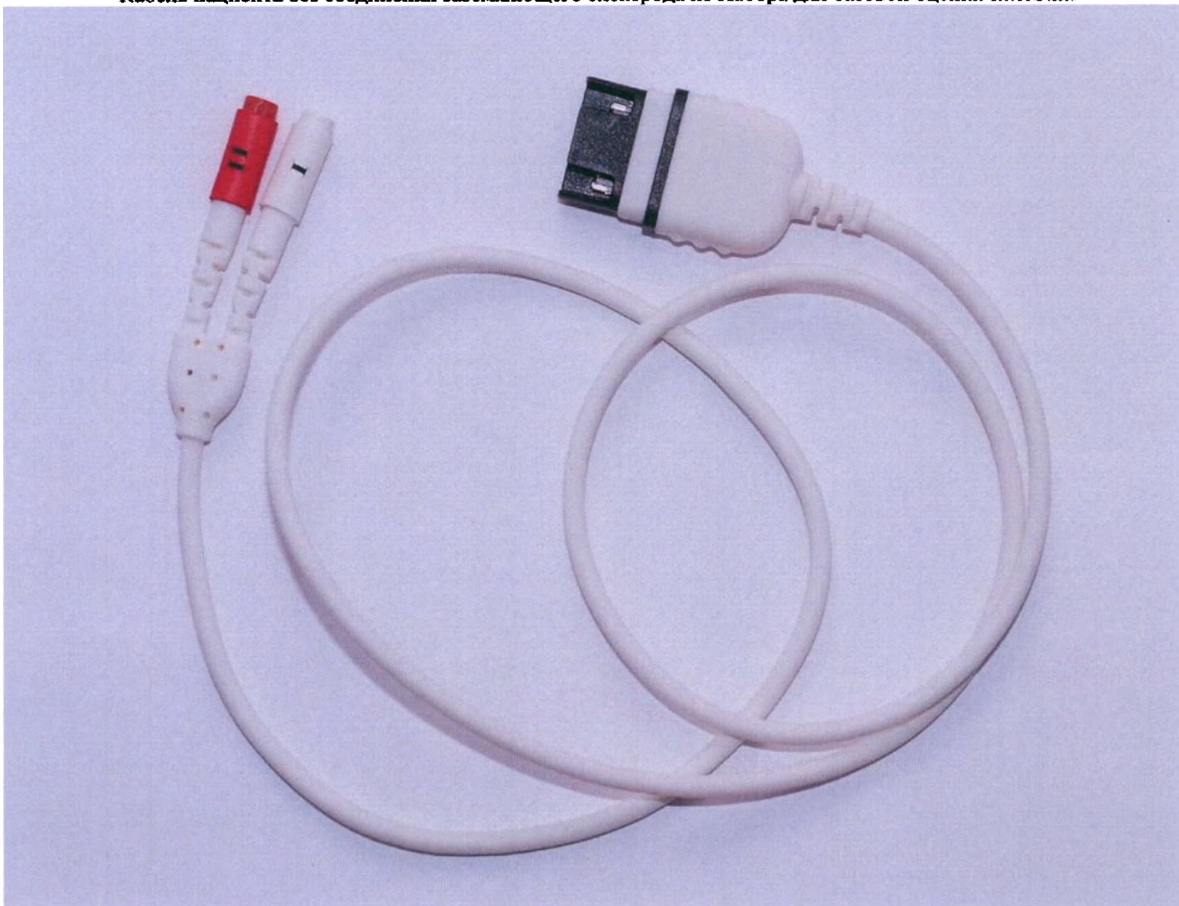
Кабель пациента без соединения заземляющего электрода из Набора для базовой оценки InterStim
