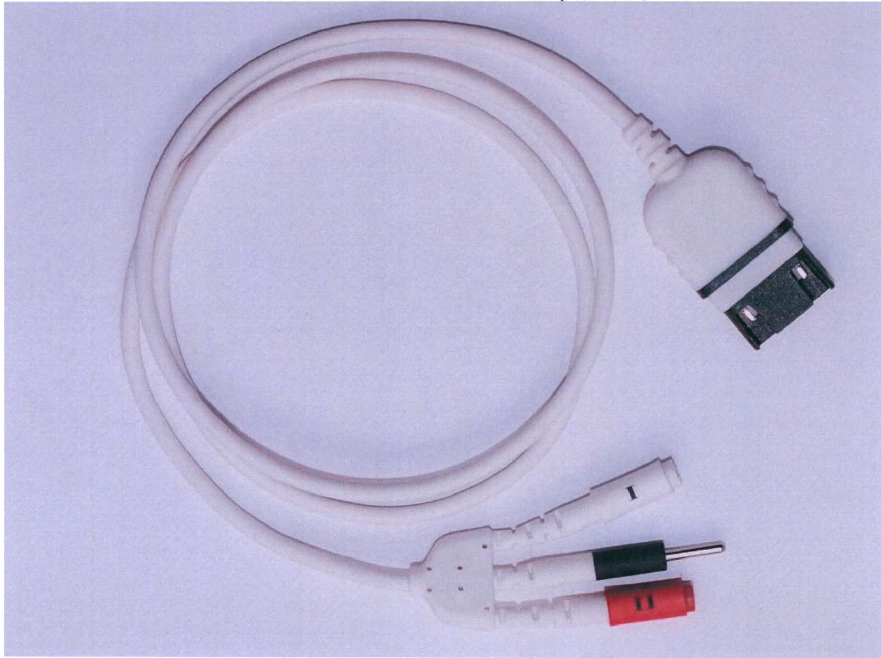
Кабель пациента с соединением заземляющего электрода: 37 см; 75 см.
