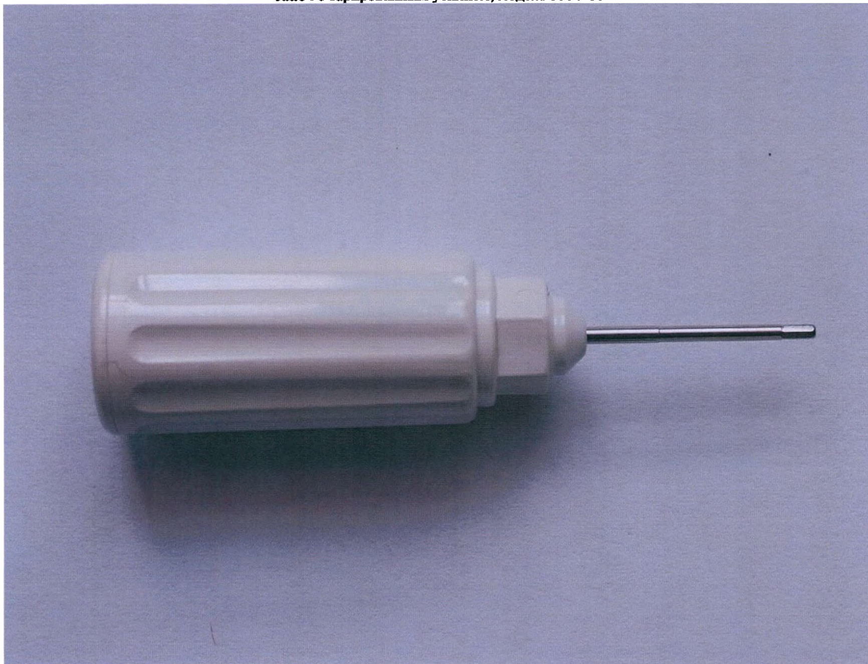
Ключ с тарированным усилием, модель 3550-80
