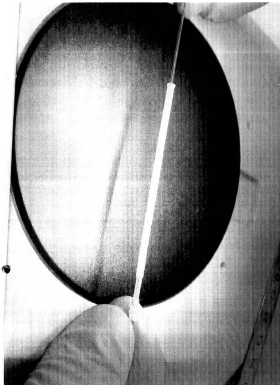
Просвет секции стента зачищается стилетом (мандреном), а внешняя поверхность покрывается защитой стента (натуральный ПТФЭ)
