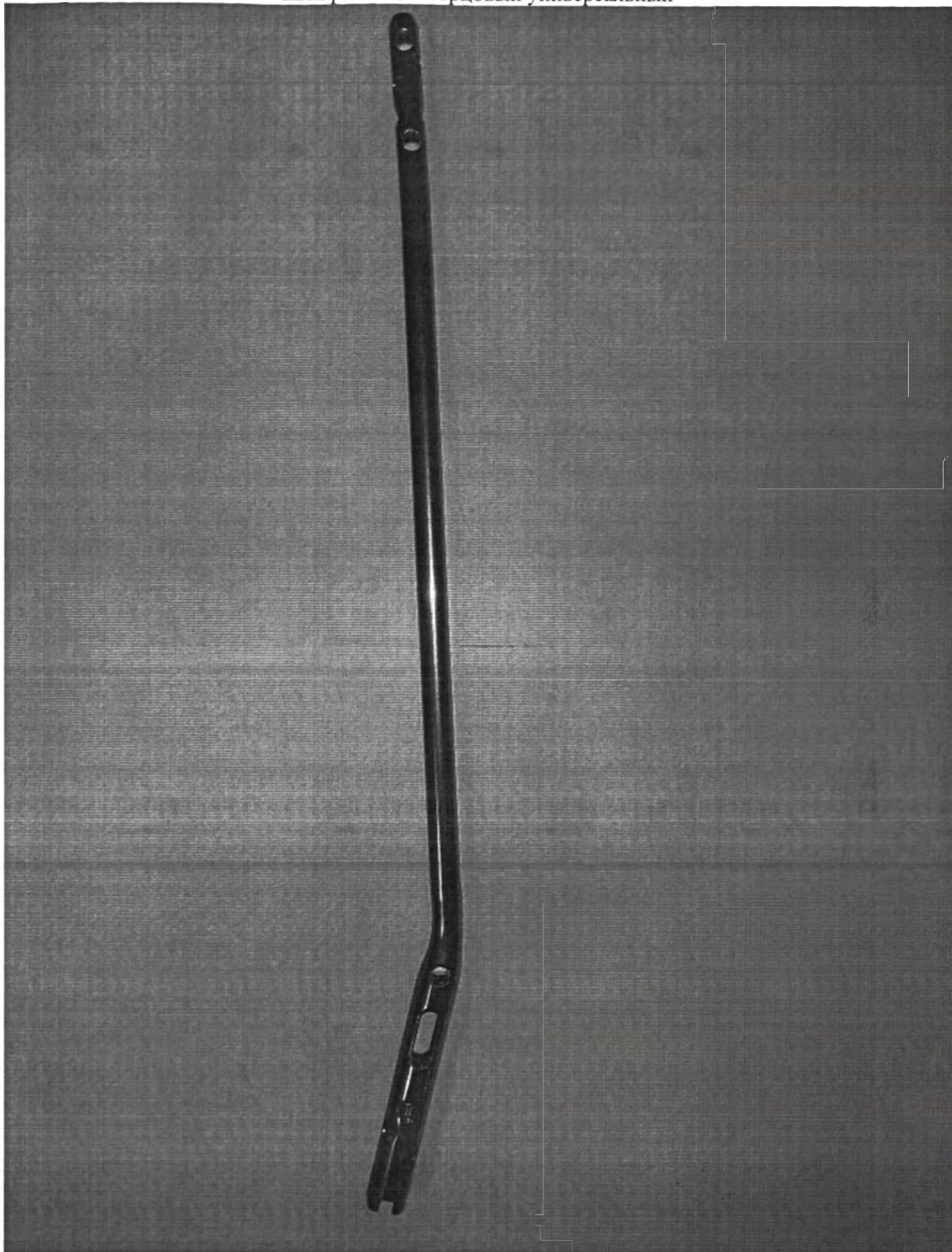
Штифт большеберцовый универсальный
