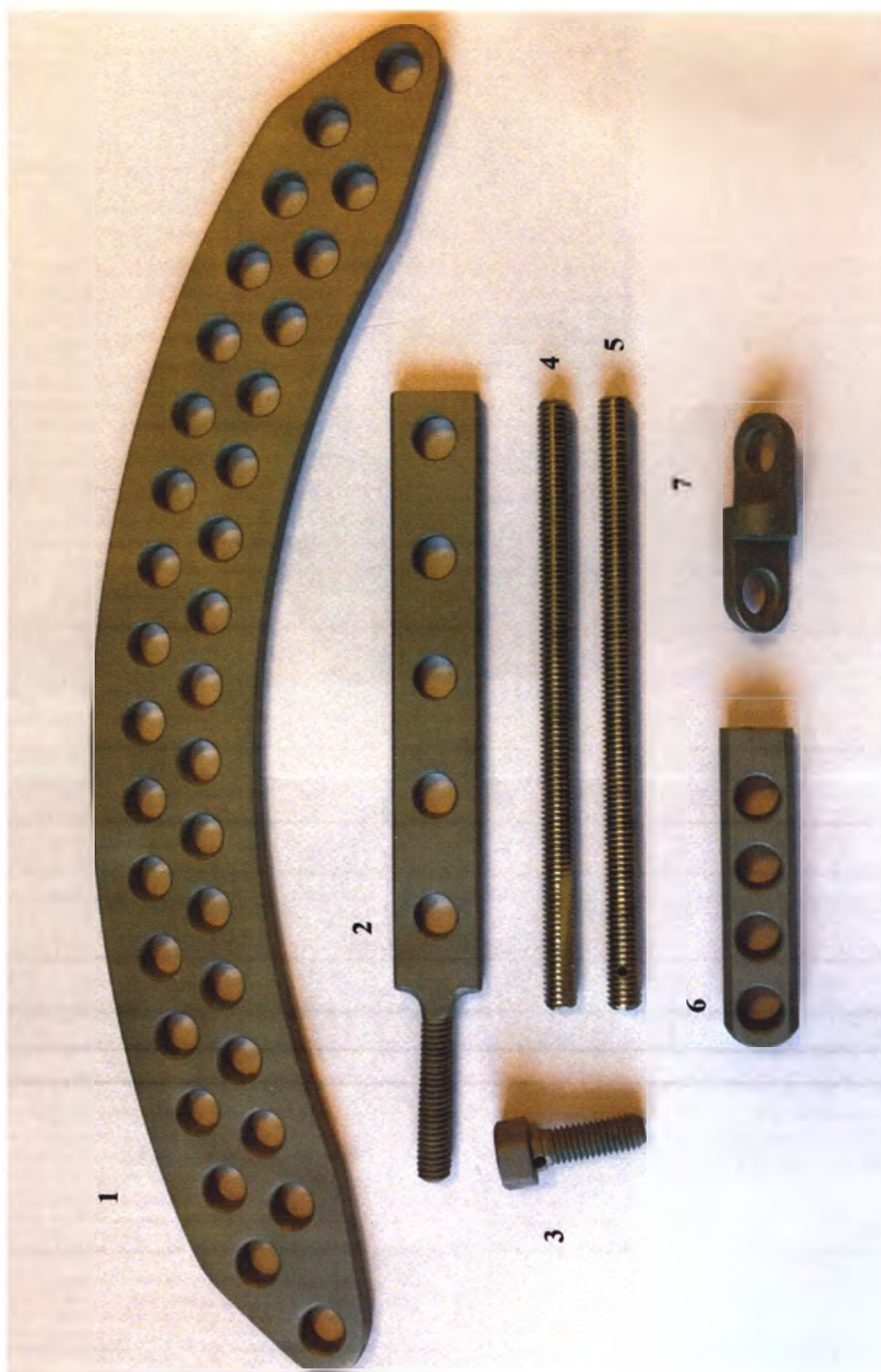
3-Общий вид медицинского изделия Комплект фиксирующих приспособлений для сборки компрессионно-дистракционных аппаратов для чрескостного остеосинтеза КфпЧО «Имплант» по ТУ 9438-001-96876955-2008
