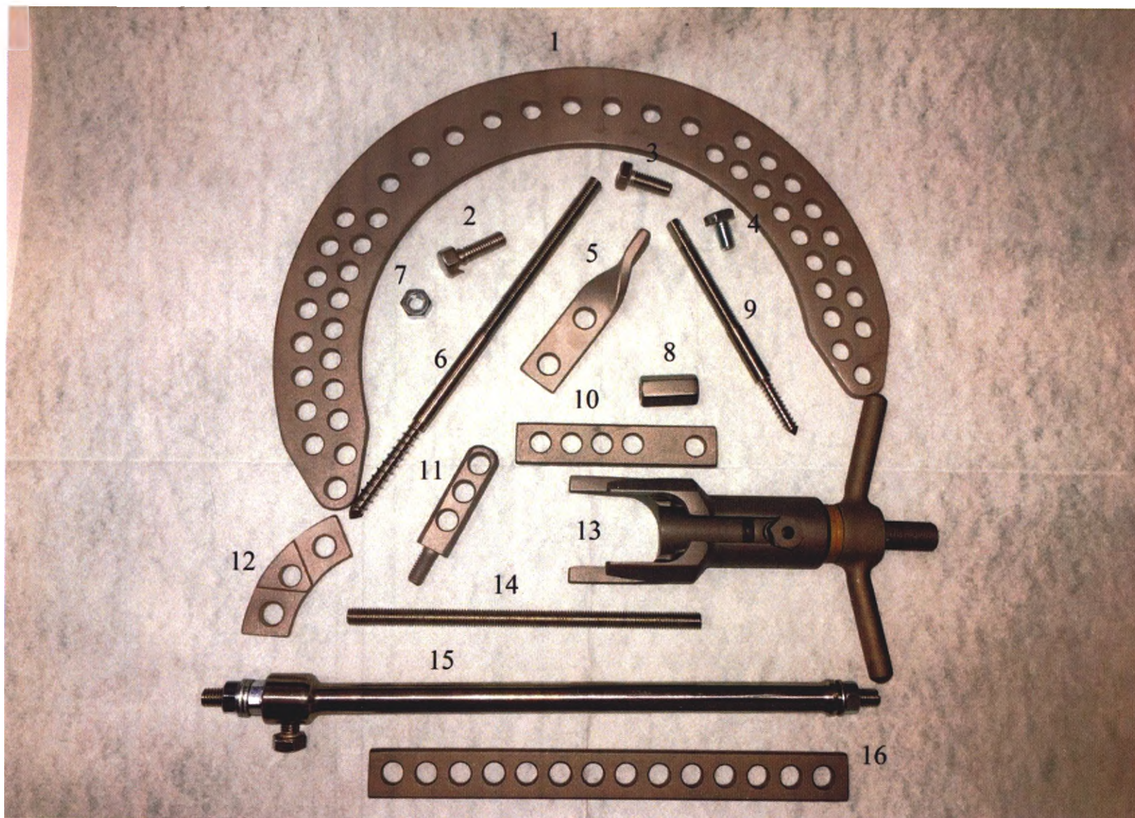
1-Общий вид медицинского изделия Комплект фиксирующих приспособлений для сборки компрессионно-дистракционных аппаратов для чрескостного остеосинтеза КфпЧО - «Имплант» по ТУ 9438-001-96876955-2008
