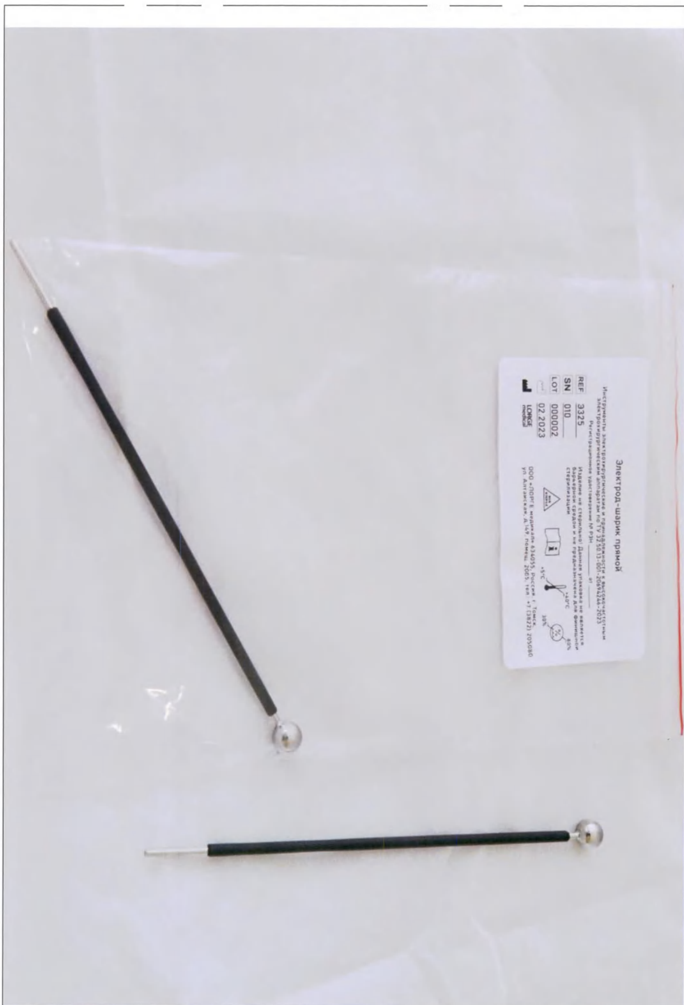
Электрод-шарик прямой Э325 – изображение общего вида изделия и изделия в индивидуальной упаковке
