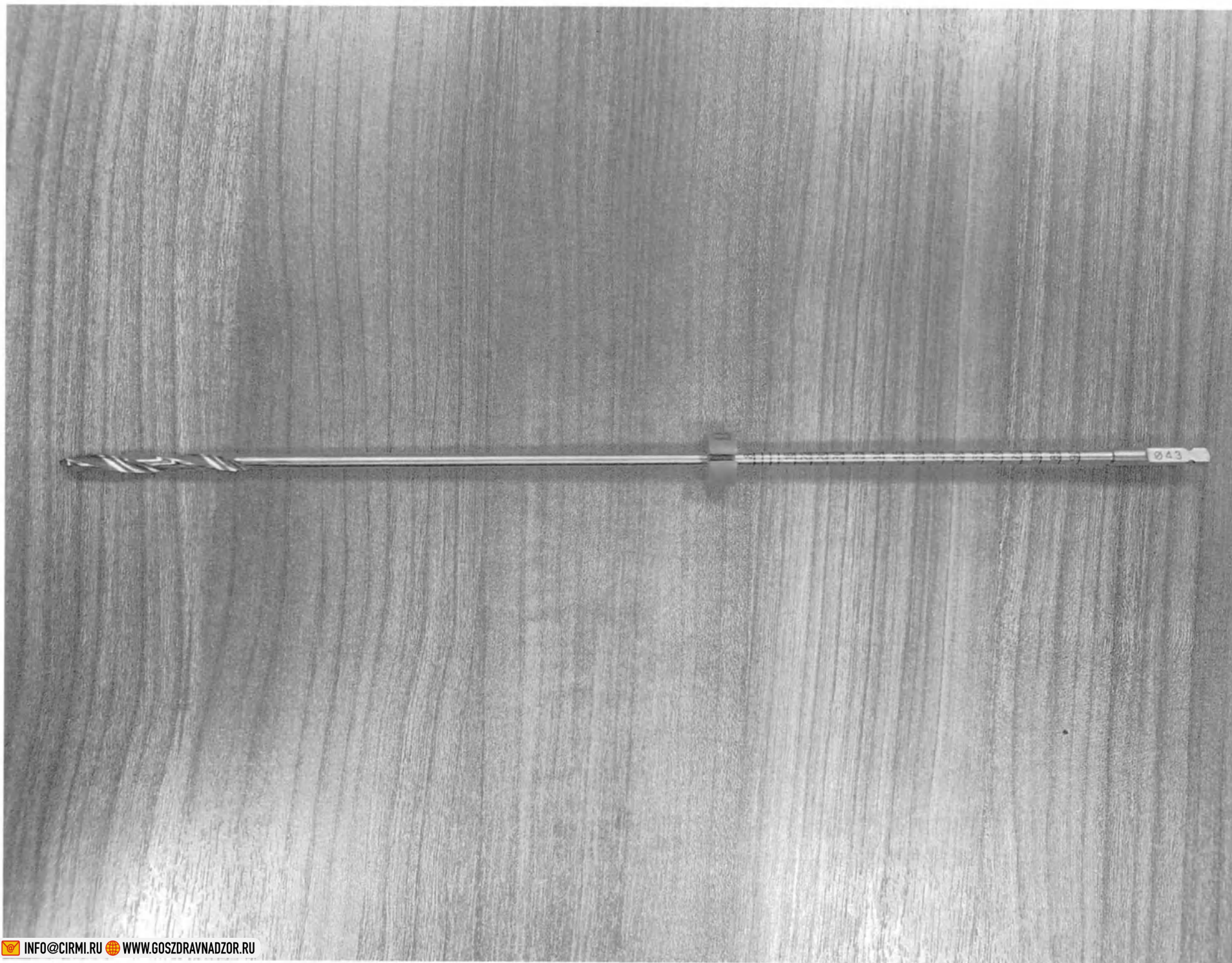
Сверло Ø 4.3 мм, длина 280 мм (общий вид)
