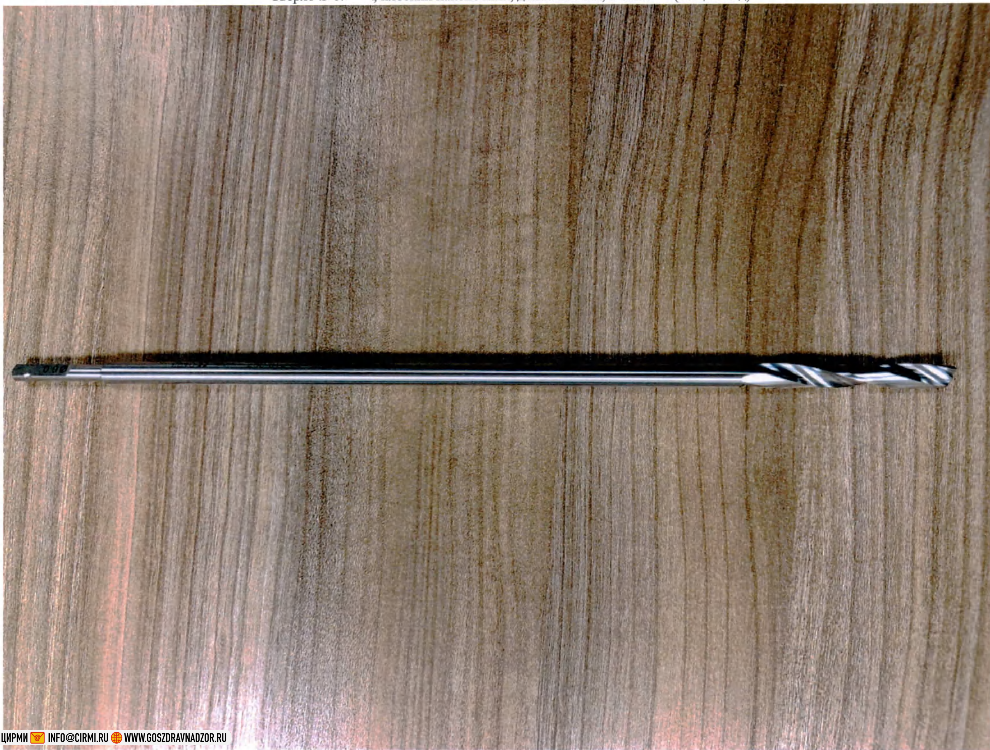
Сверло Ø 6.1, плоский наконечник, длина 250 мм, 2 канала (общий вид)
