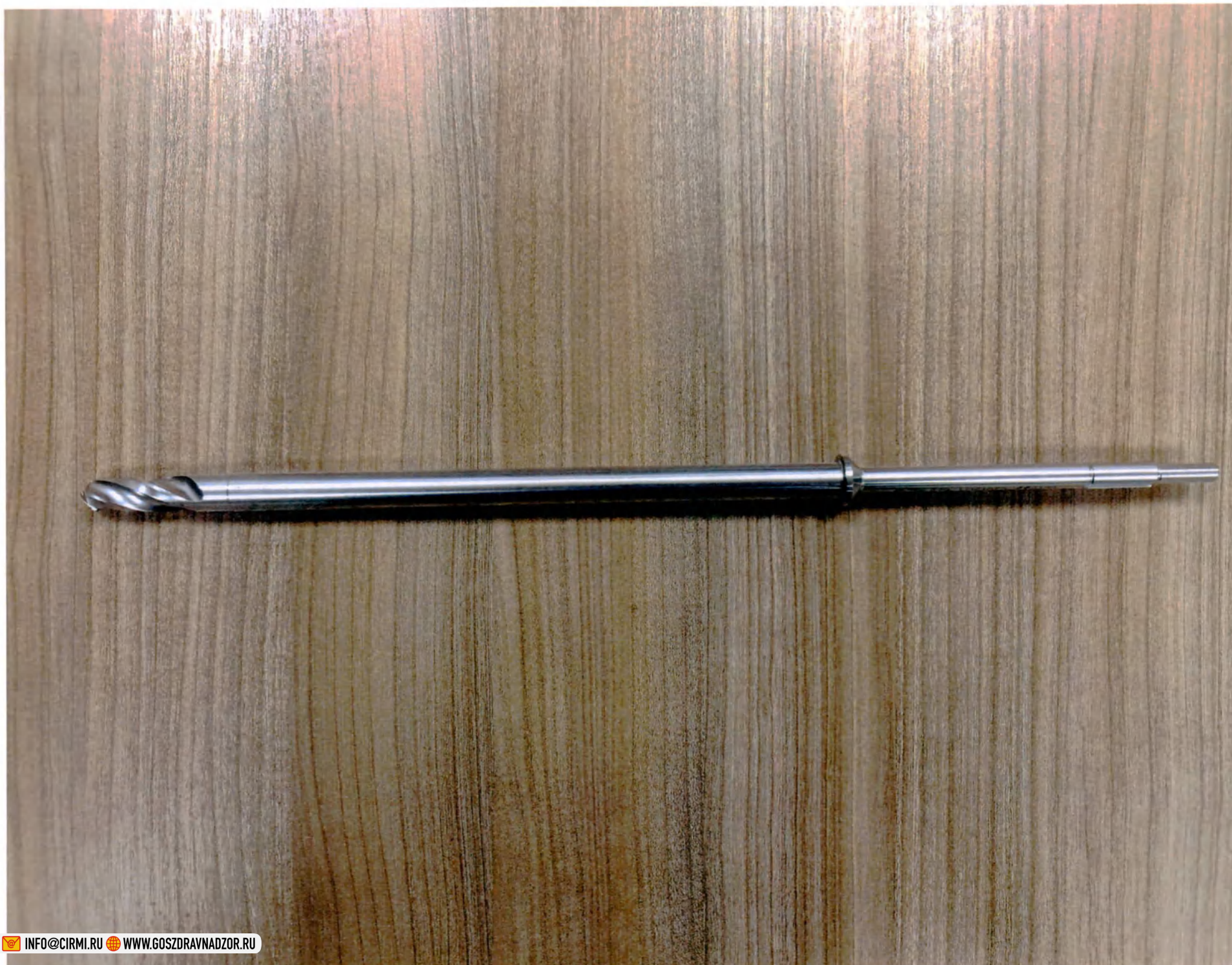
Сверло Ø 11.0 мм, длина 354 мм (общий вид)
