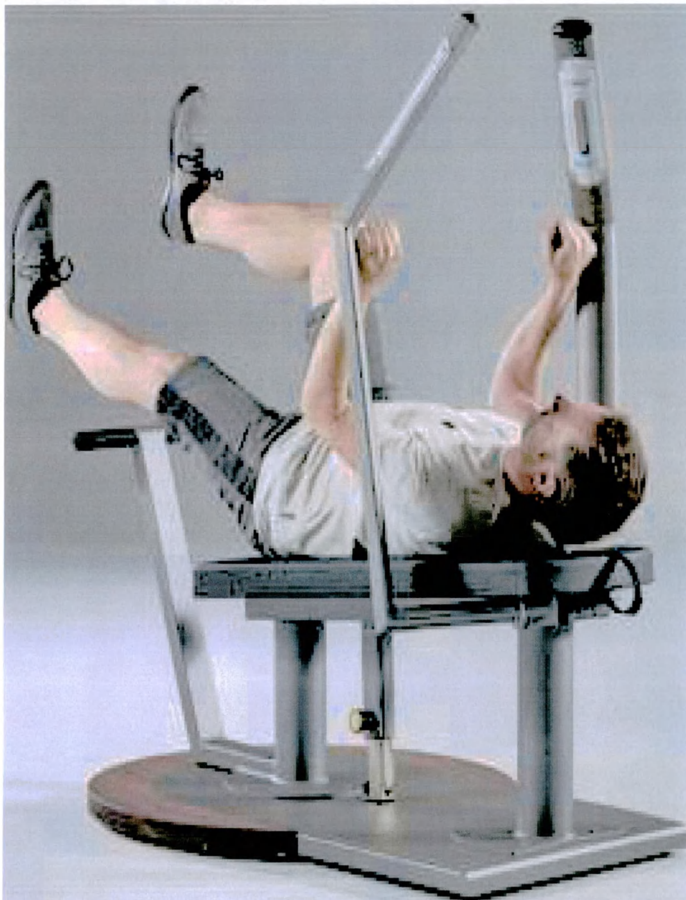
Рисунок 5.2. Устройство Transversus-Trainer 917
