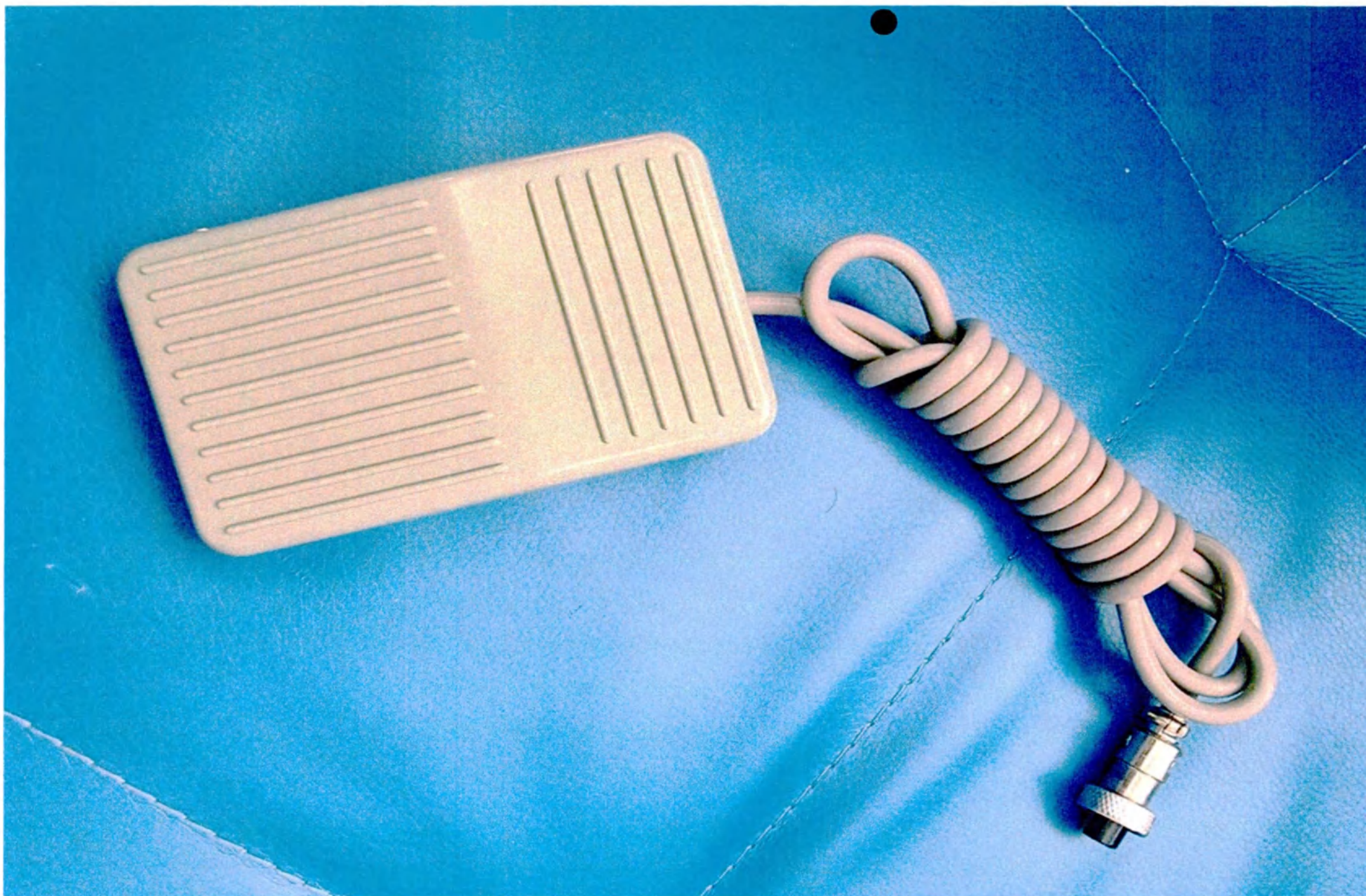
Рисунок 6.9 - Ножной выключатель
