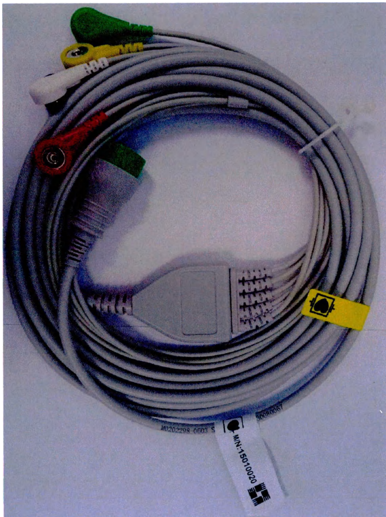
Кабель ЭКГ для взрослых/детей. Общий вид
