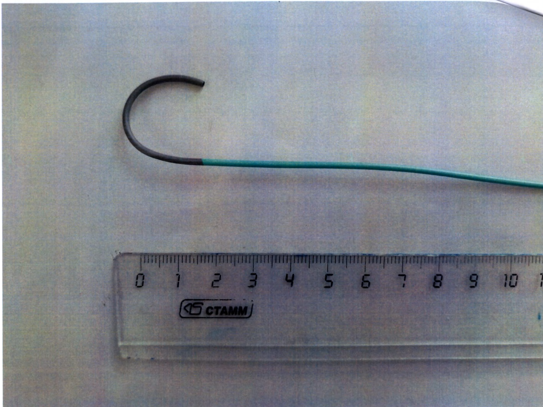
Кончик типа RC2
