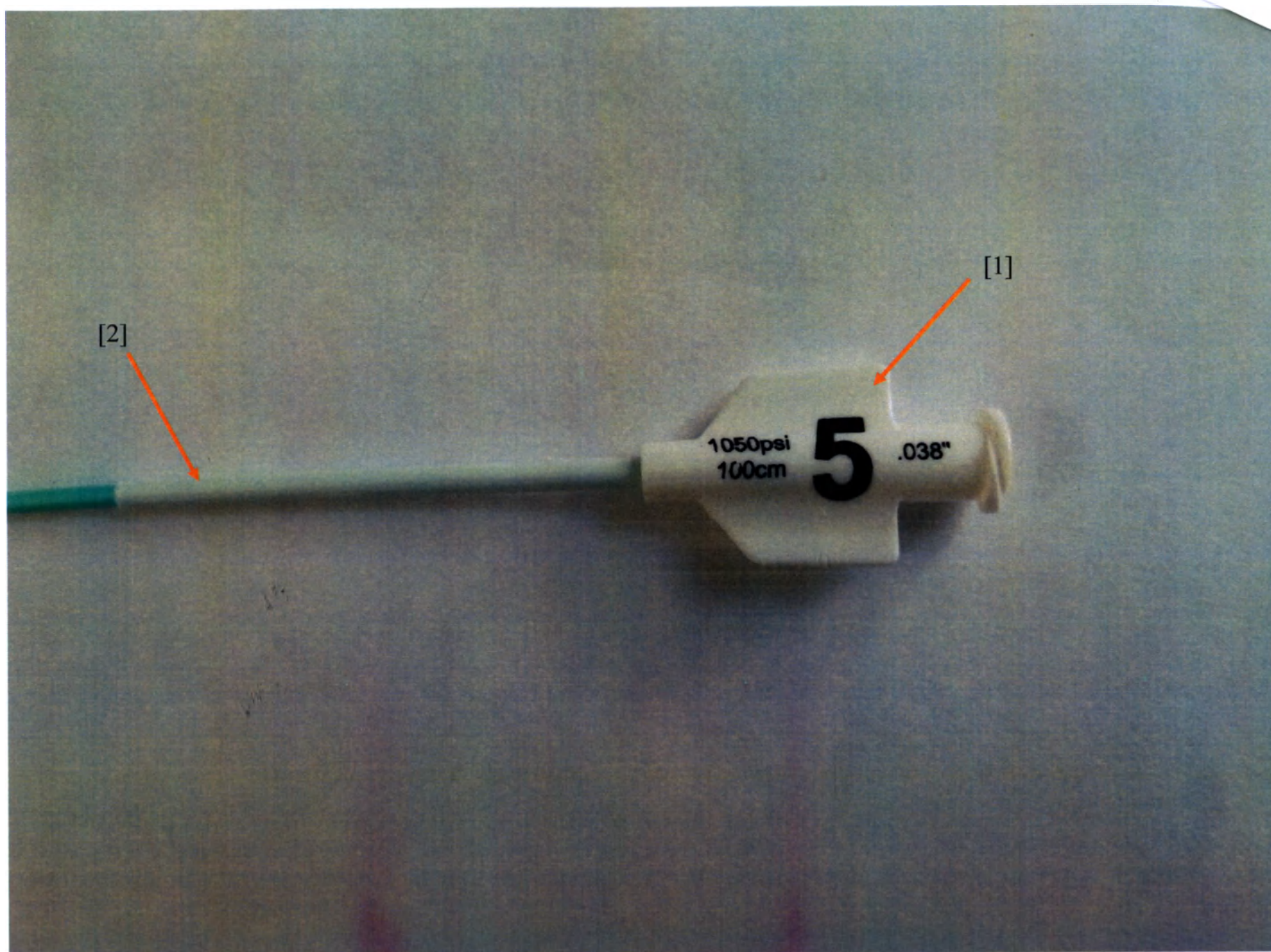
Хаб [1] и разгрузочная муфта [2]
