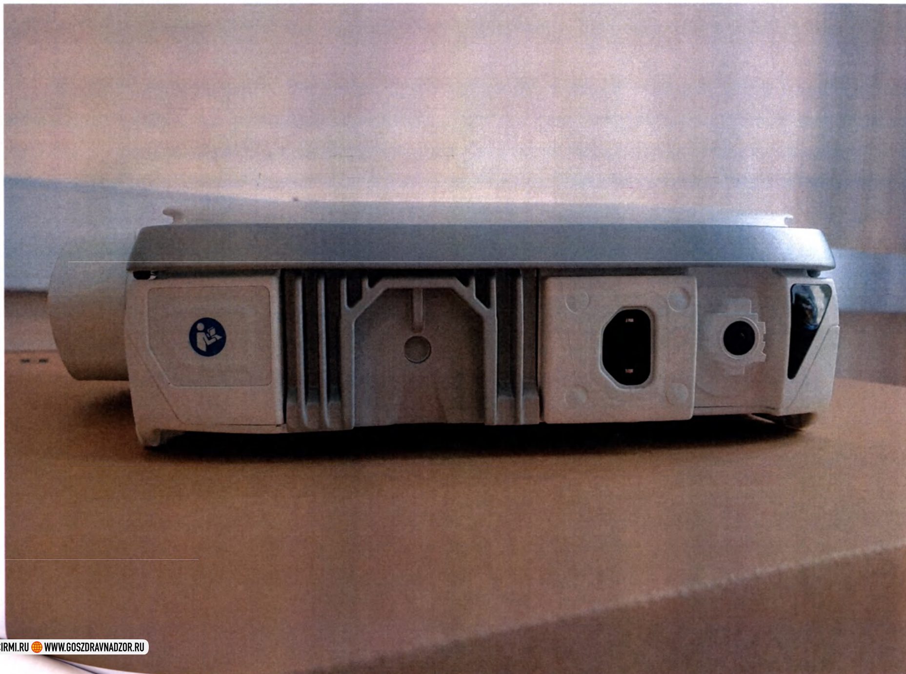
Насос инфузионный шприцевой «Перфузор® Спэйс плюс» (Spaceplus Perfusor®) арт. № 8719030, вид сзади
