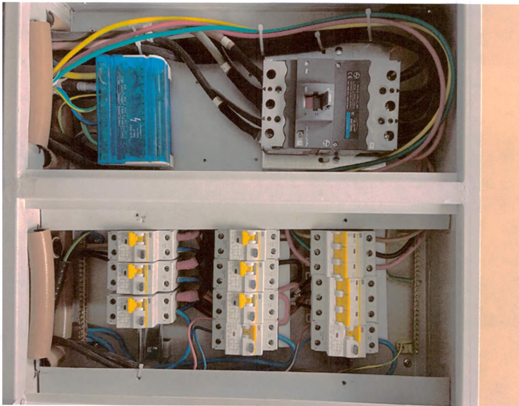
Щит распределительный
