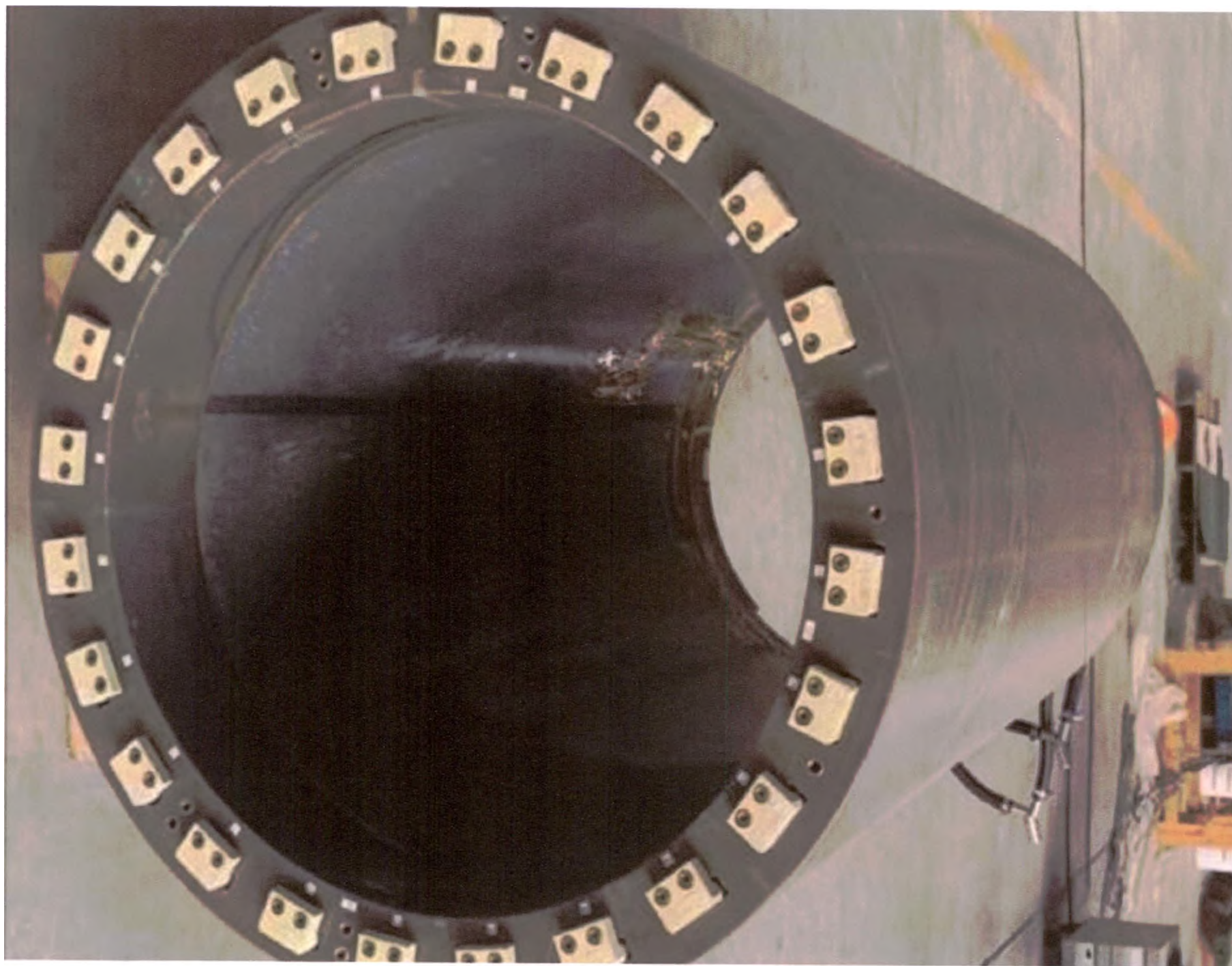
Градиентная катушка
