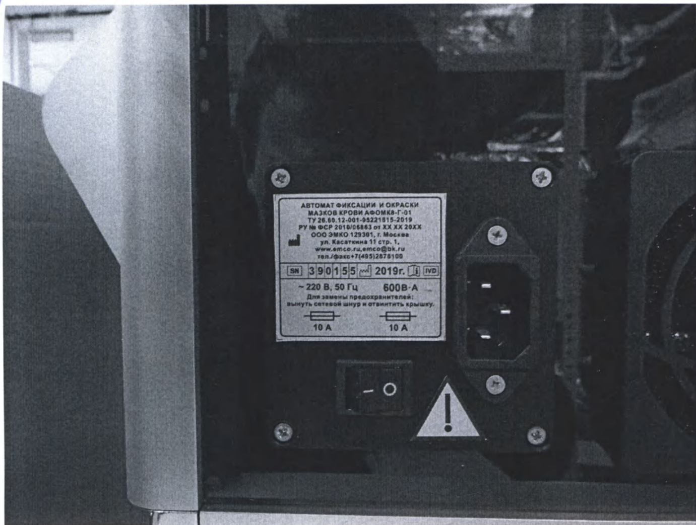
АФОМК8-Г-01 (маркировка)
