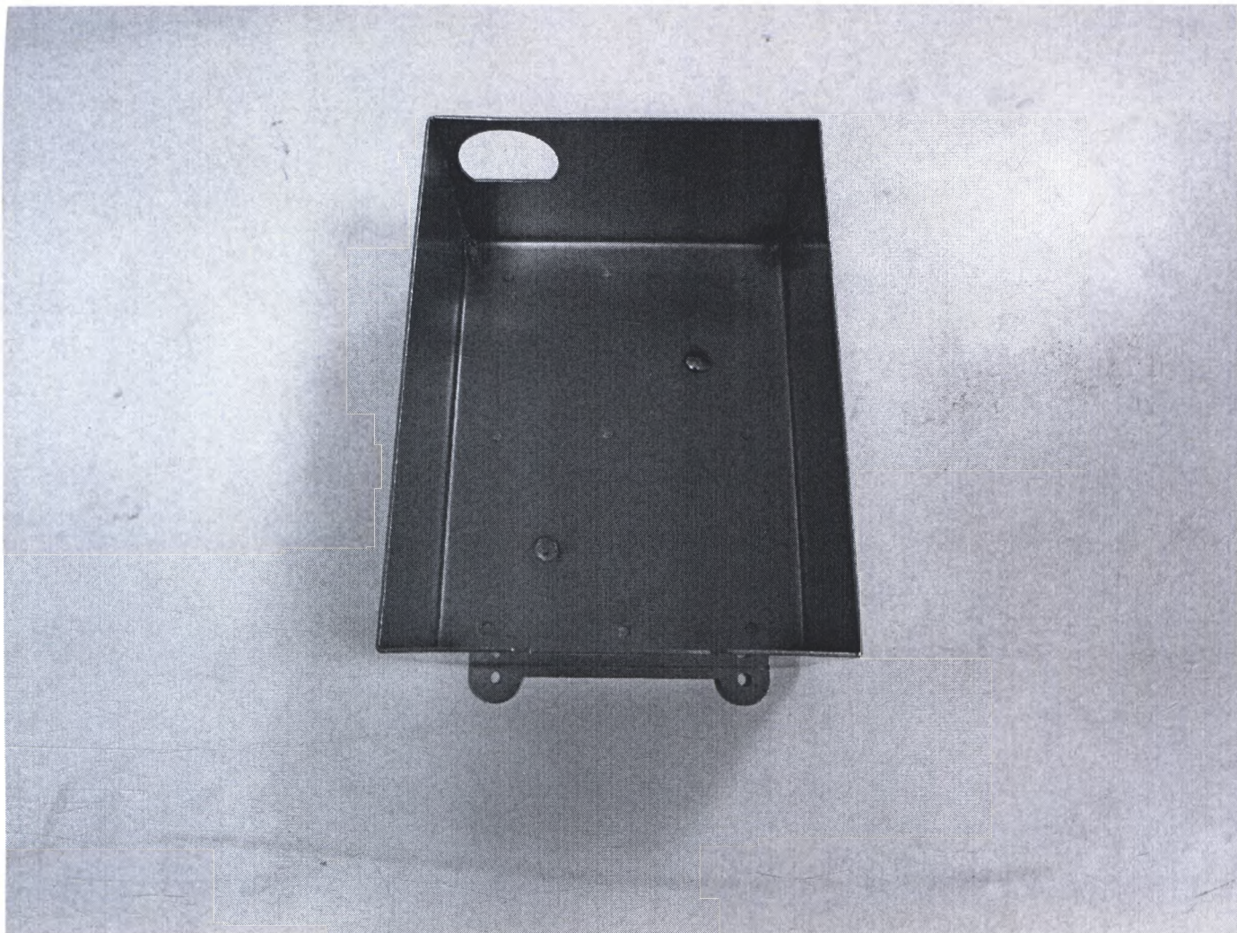
Ванна проточная-Г8
