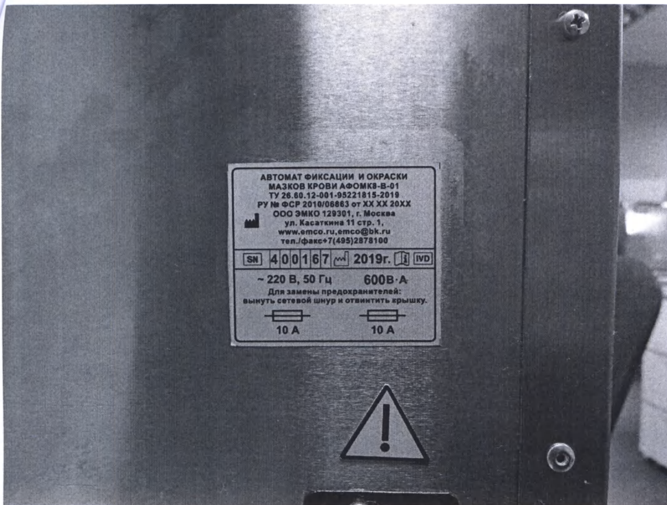
АФОМК8-В-01 (маркировка)
