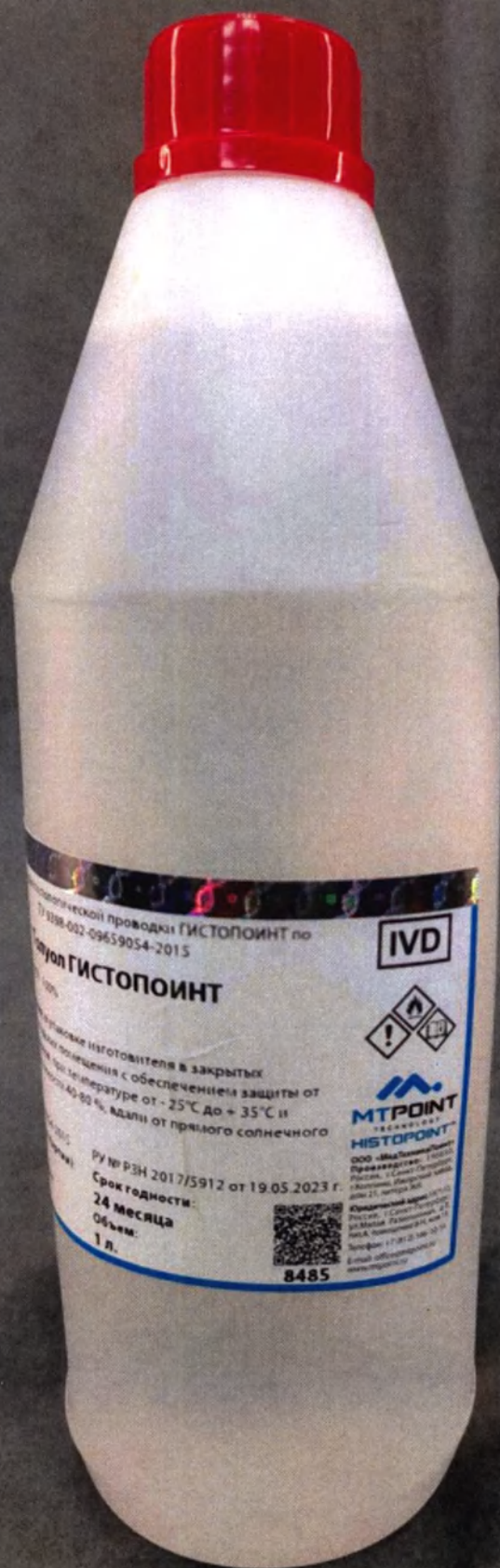
5.3 Толуол
