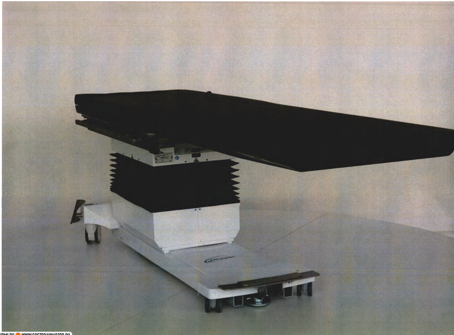
Стол рентгенохирургический Медин-Сафис с принадлежностями (ПУ № РЗН 2018/6853) Общий вид
