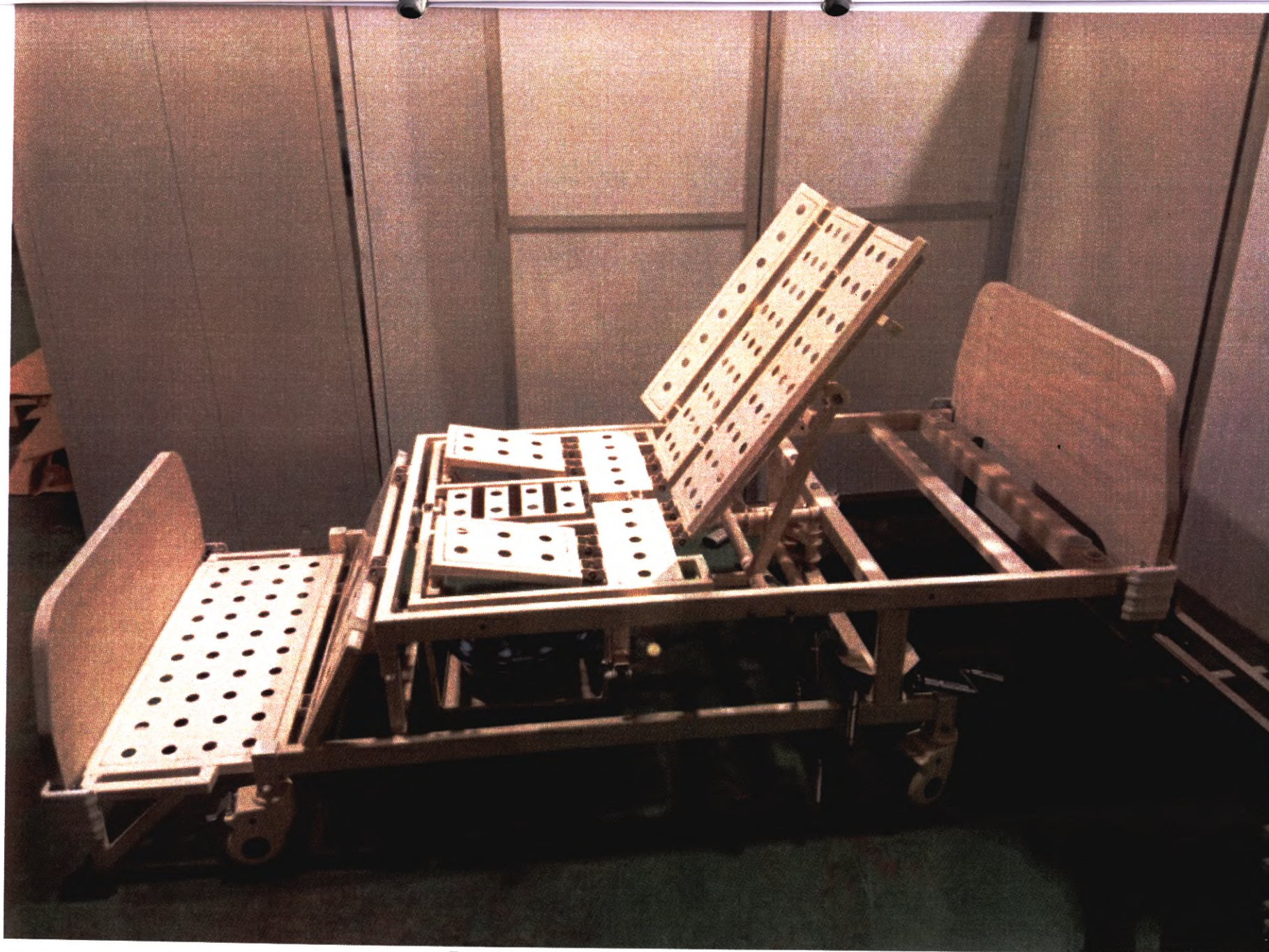
Рис.1.4. Сидячее положение, вид сбоку.
