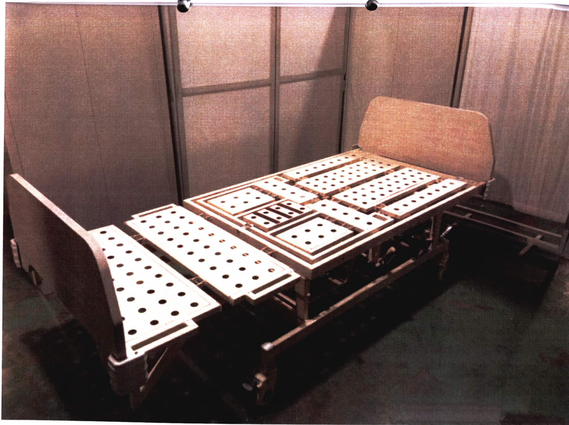
Рис. 1.2. Горизонтальное положение, вид в аксонометрии.
