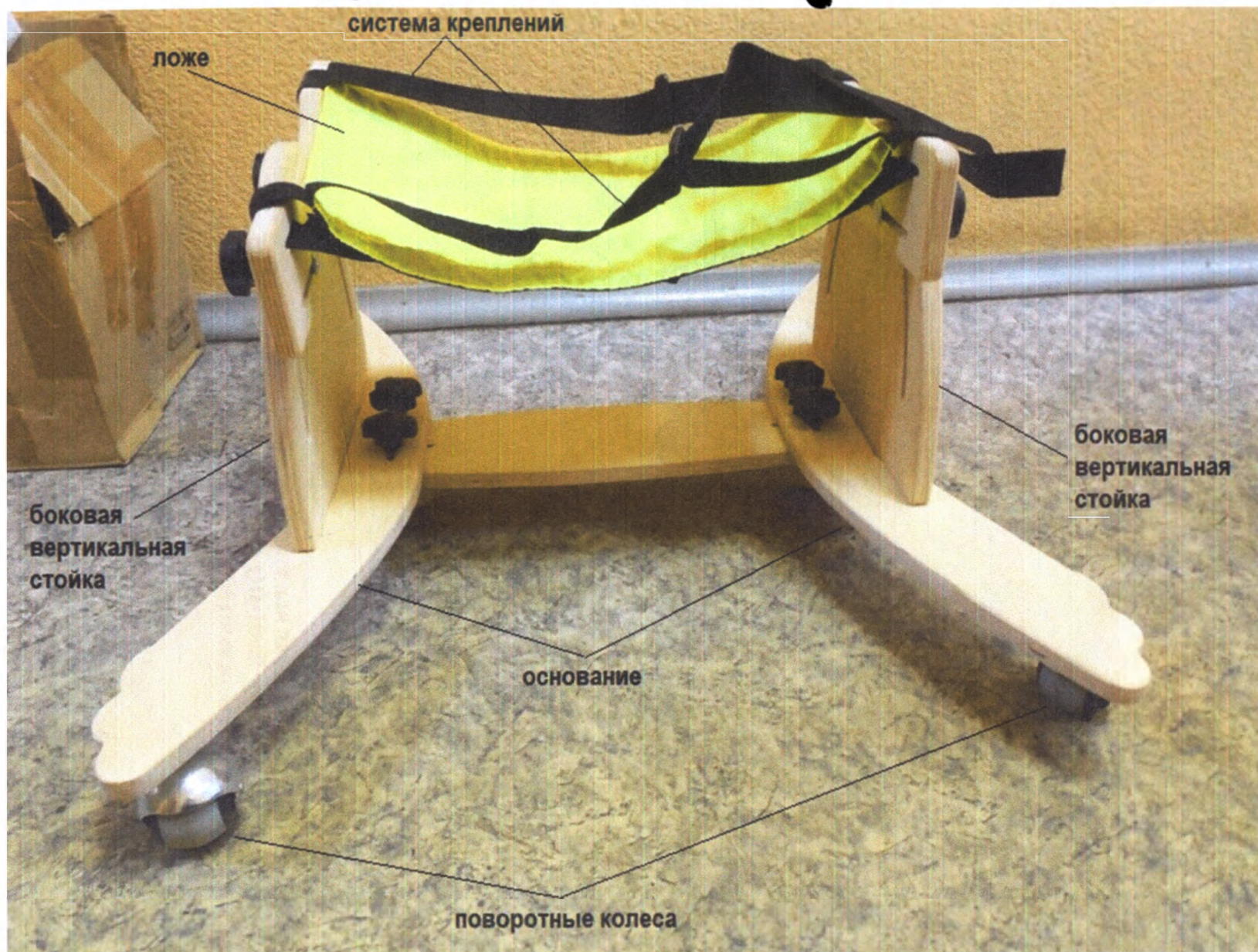
1-Опора функциональная для ползания для детей-инвалидов «Я МОГУ!», исполнение ОП-109.1
