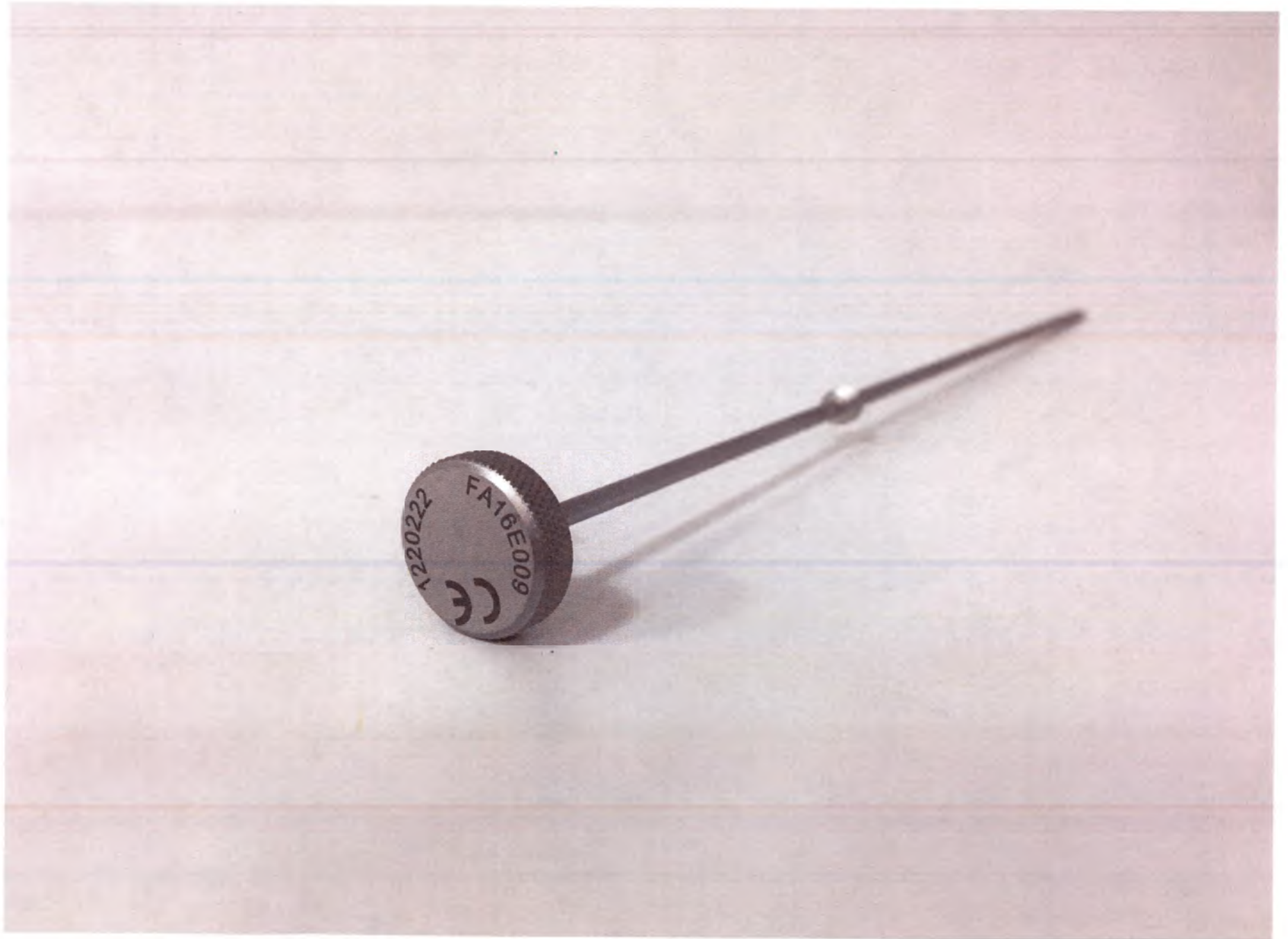
Вал установителя кейджа, резьбовой.
