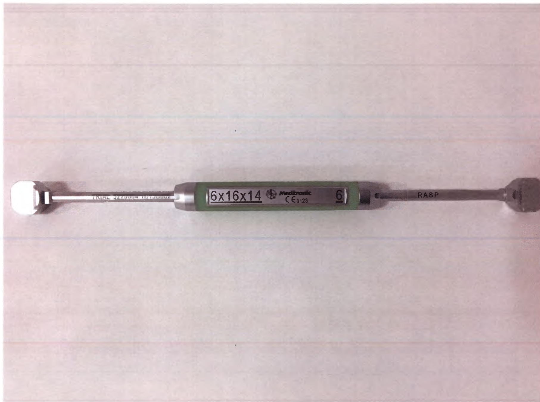
Рашпиль, 16 мм х 14 мм х 6 мм.
