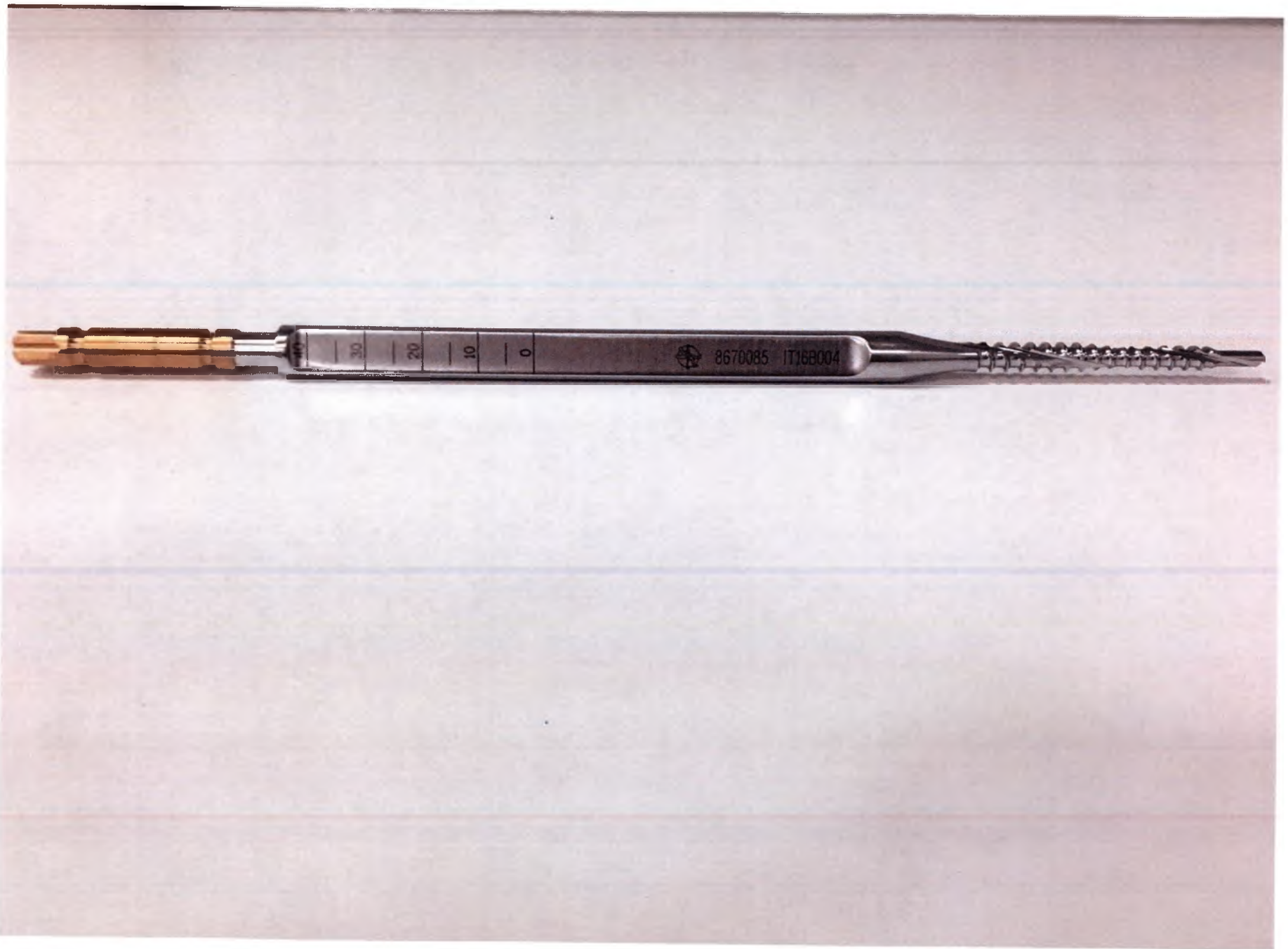
Метчик канюлированный, саморезный, 4,5-5,5 мм.
