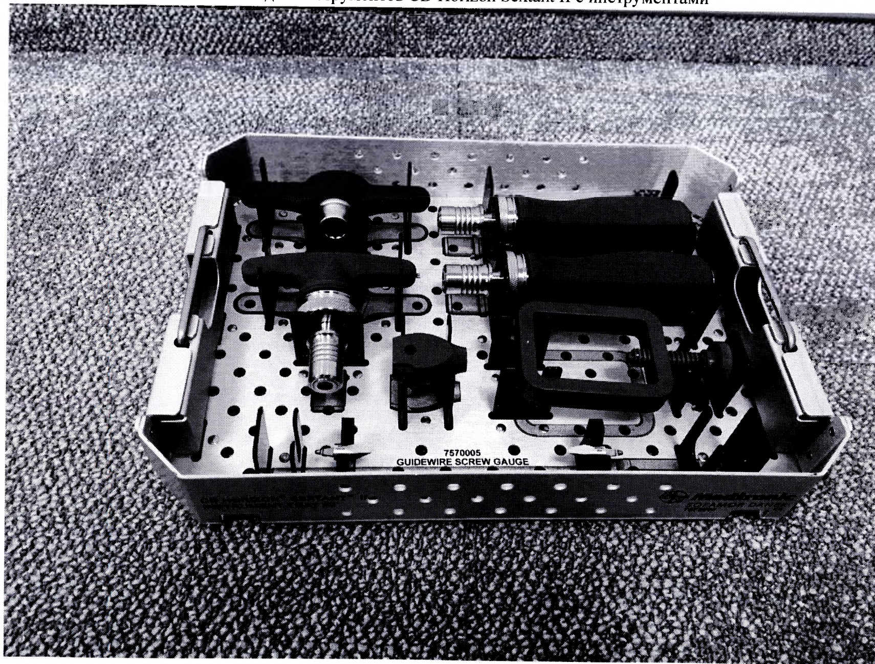
Полка №2 для инструментов CD Horizon Sextant II с инструментами
