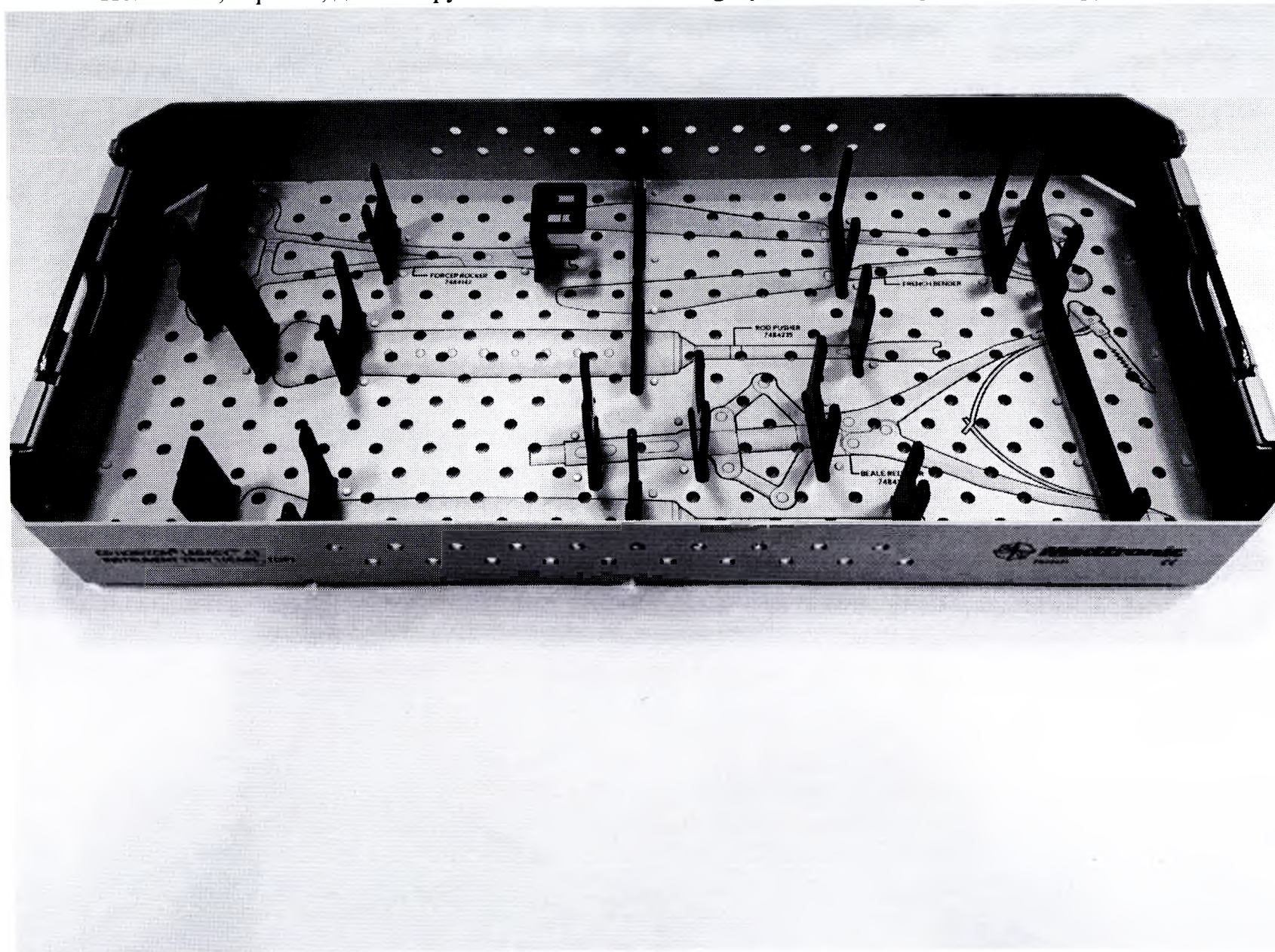
Полка №1, верхняя, для инструментов CD Horizon Legacy 4.5, контейнер №1 без инструментов
