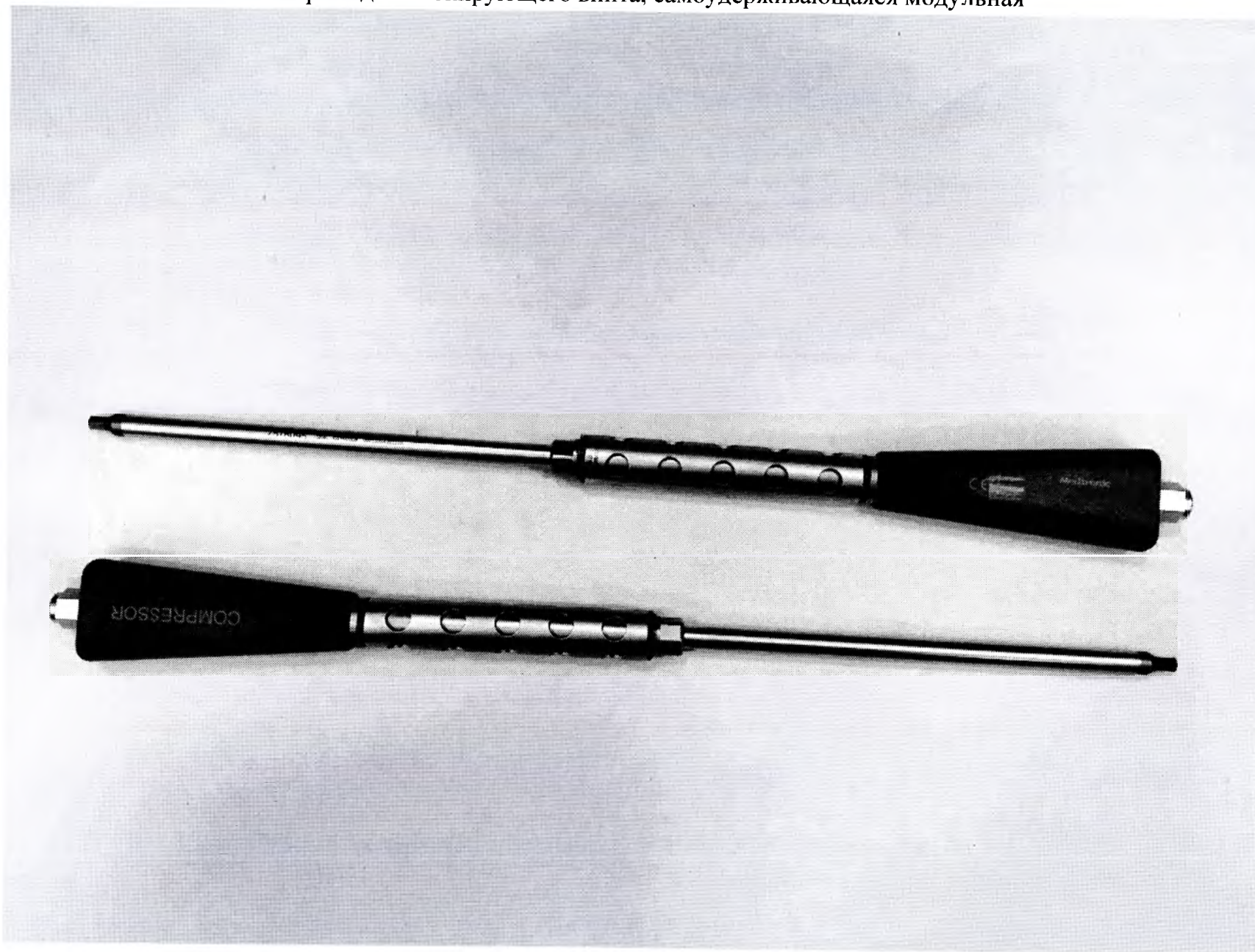
Отвертка для блокирующего винта, самоудерживающаяся модульная
