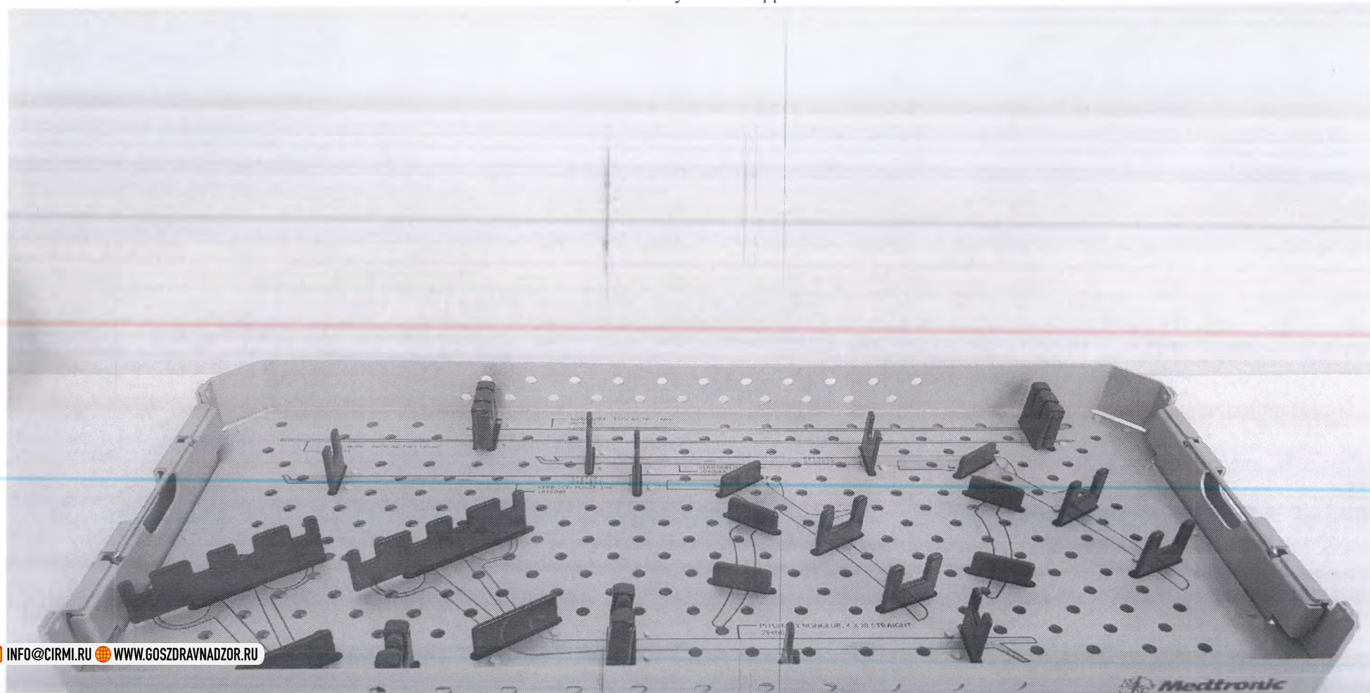
- Полка для кусачек Керрисона
