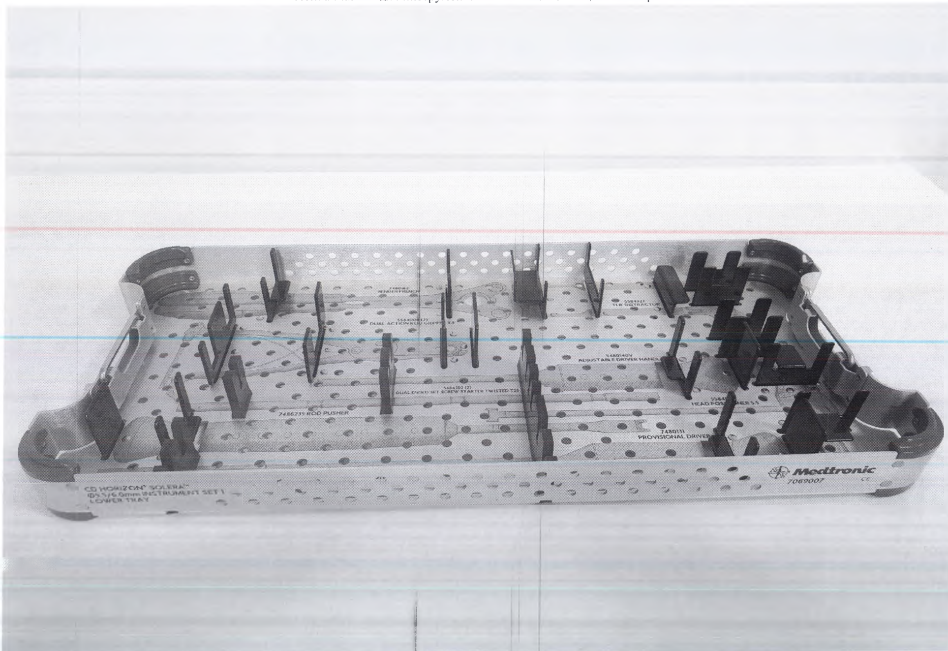
- Полка нижняя для инструментов CD Horizon Solera, контейнер №1
