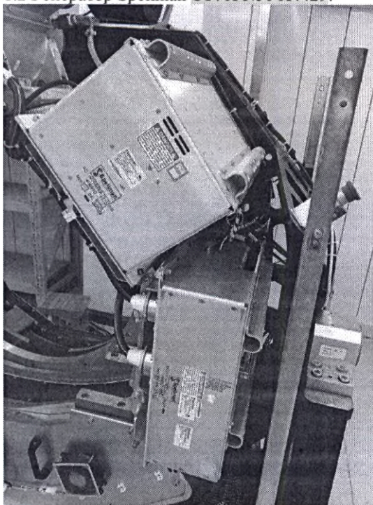
1.3 Излучатель рентгеновский с трубкой CTR 2280CESV.
