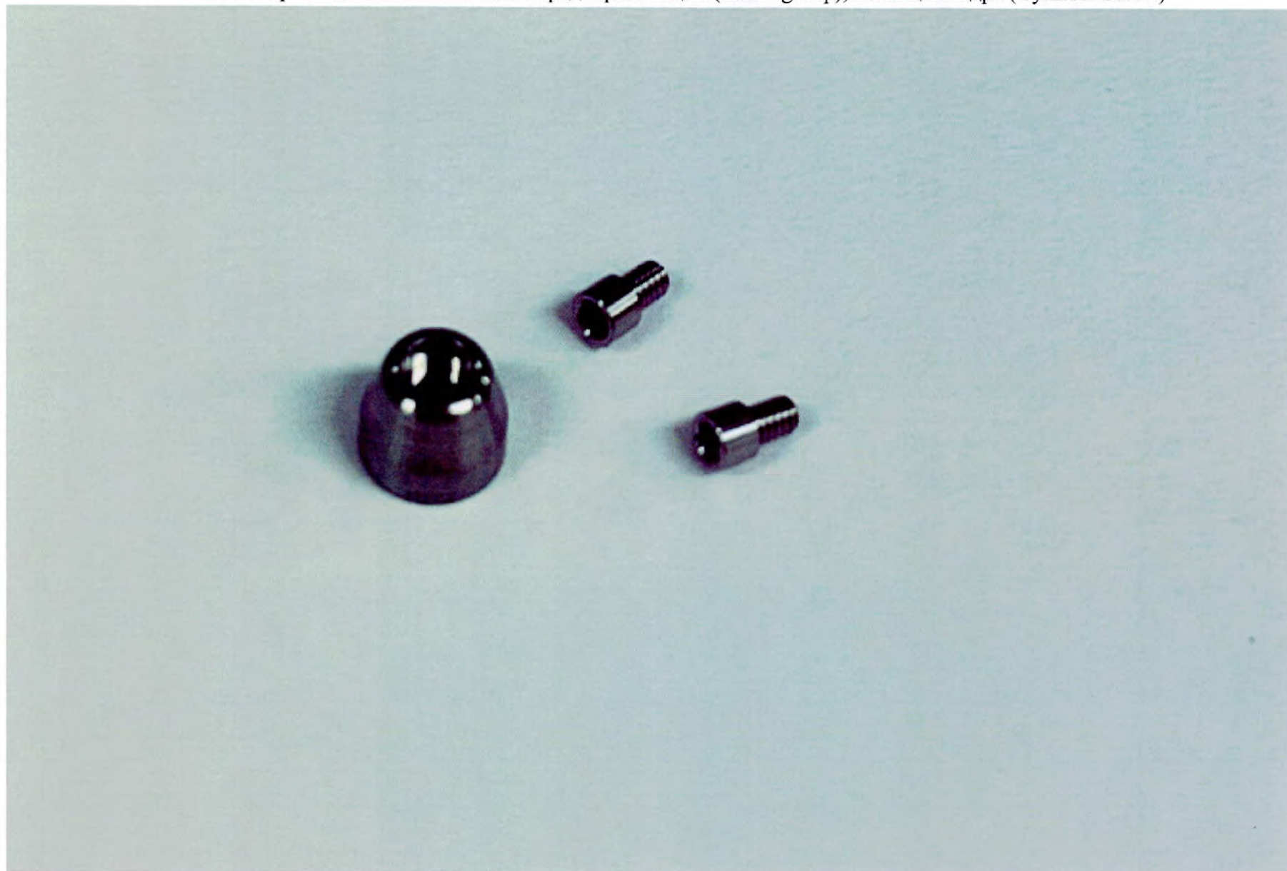
Компоненты ортопедические: Колпачок предохраняющий (Healing Cap), Винт цилиндра (Cylinder Screw)
