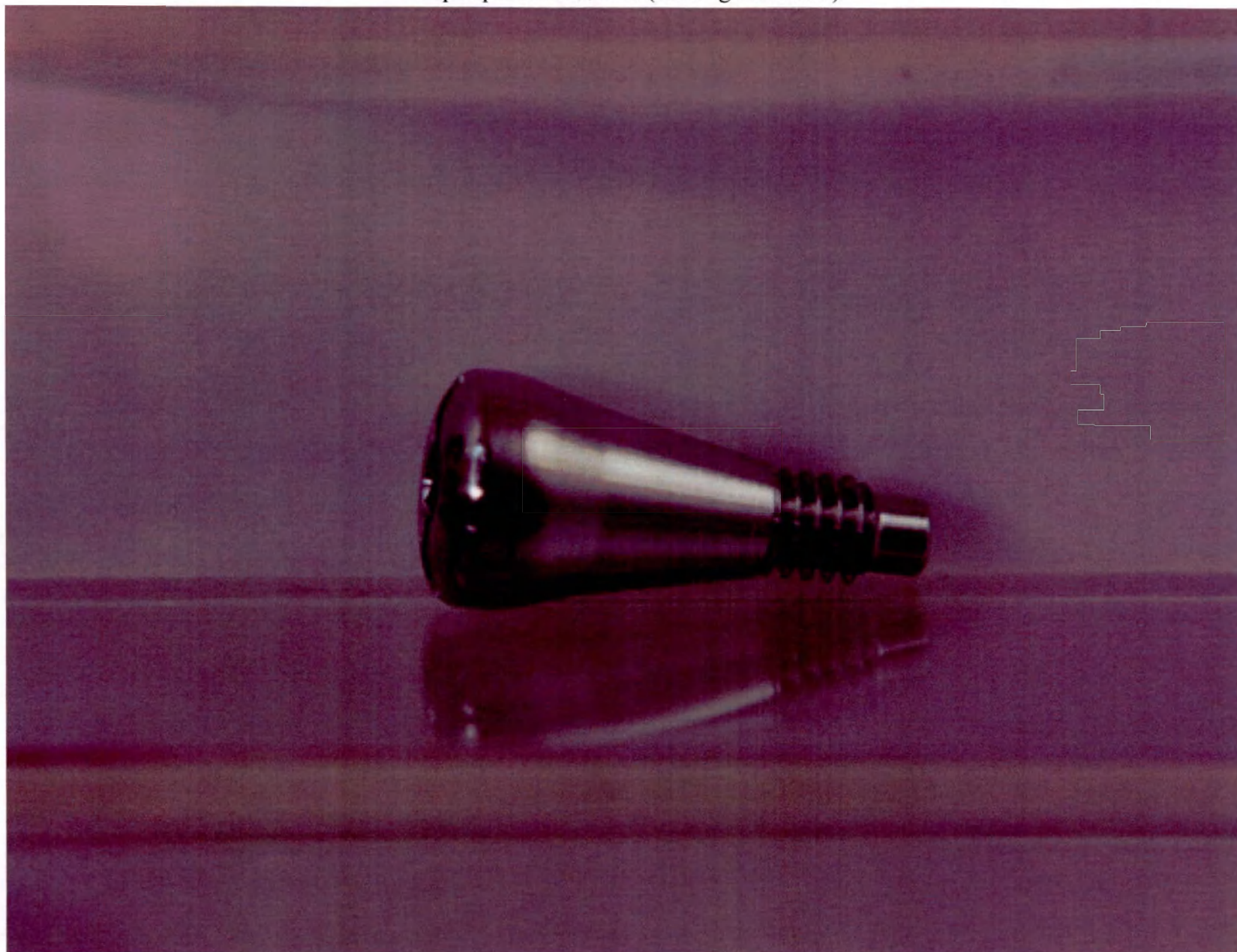
Формирователь десны (Healing Abutment)
