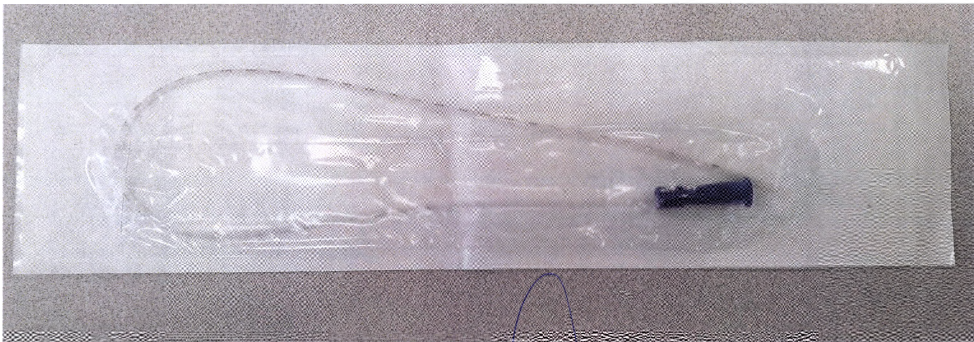
Фото 1 – Медицинское изделие 13032185 Катетер Мюлли метрический с воронкообразным коннектором в бумажно-пленочной упаковке по ГОСТ ISO 11867-1
