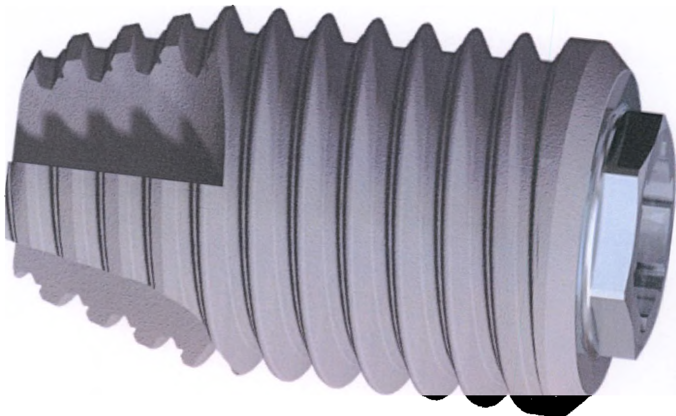
Натяжной NobelSpeedy® Groovy WP 6x10 mm
