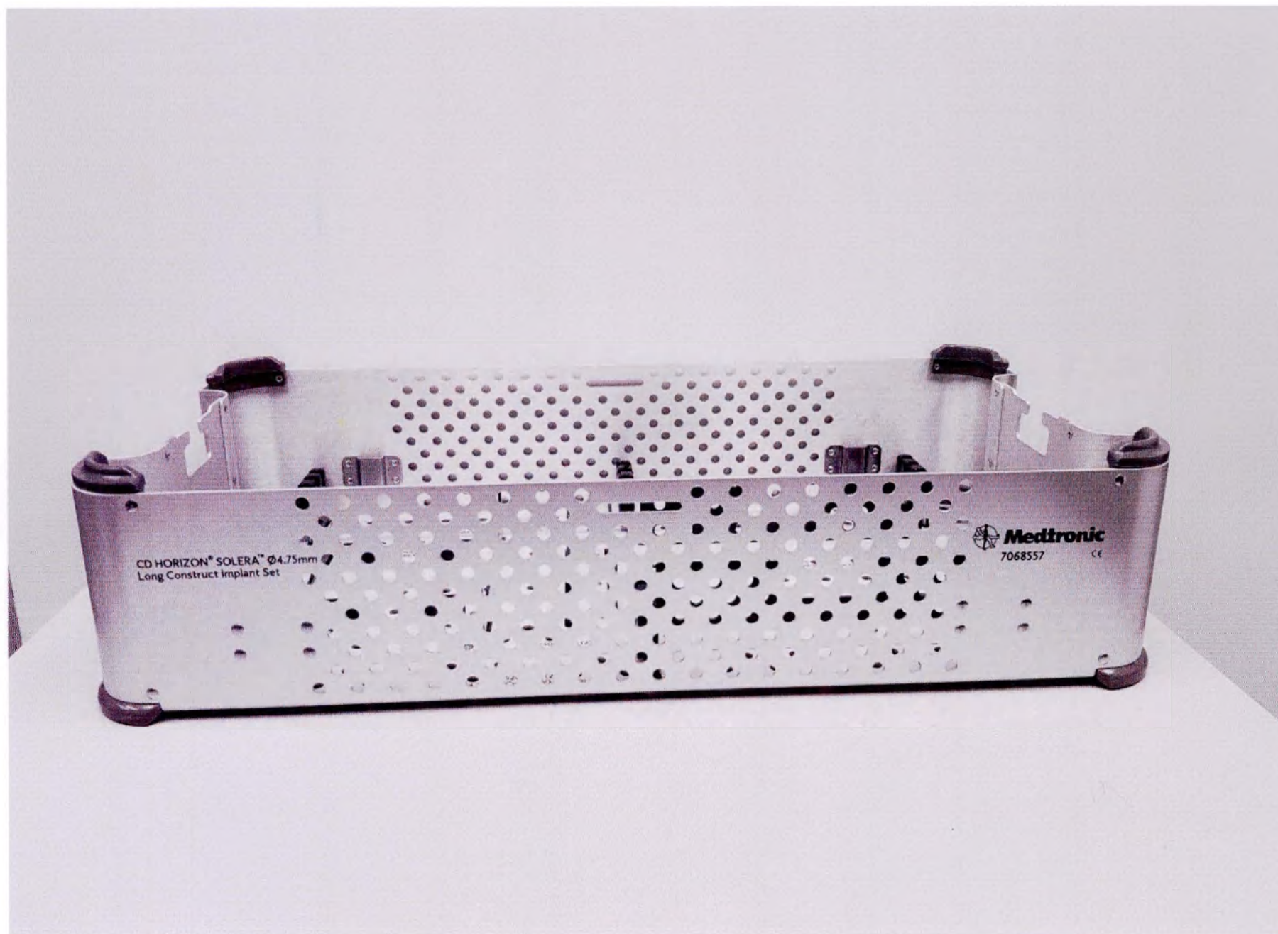
Полка нижняя 4,75 мм
