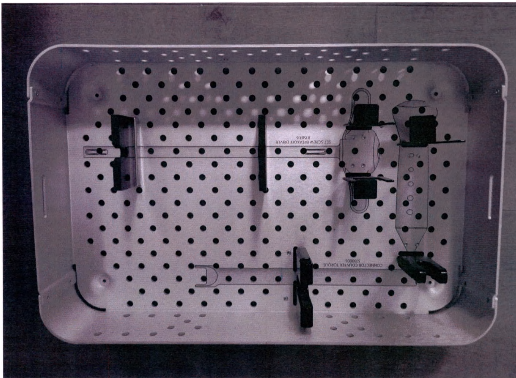
Контейнер для инструментов установки коннекторов с изменяемым углом
