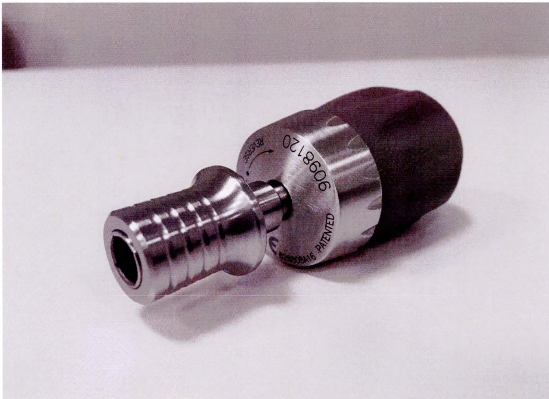
Рукоятка канюлированная яйцевидная "с трещоткой" для сменных инструментов
