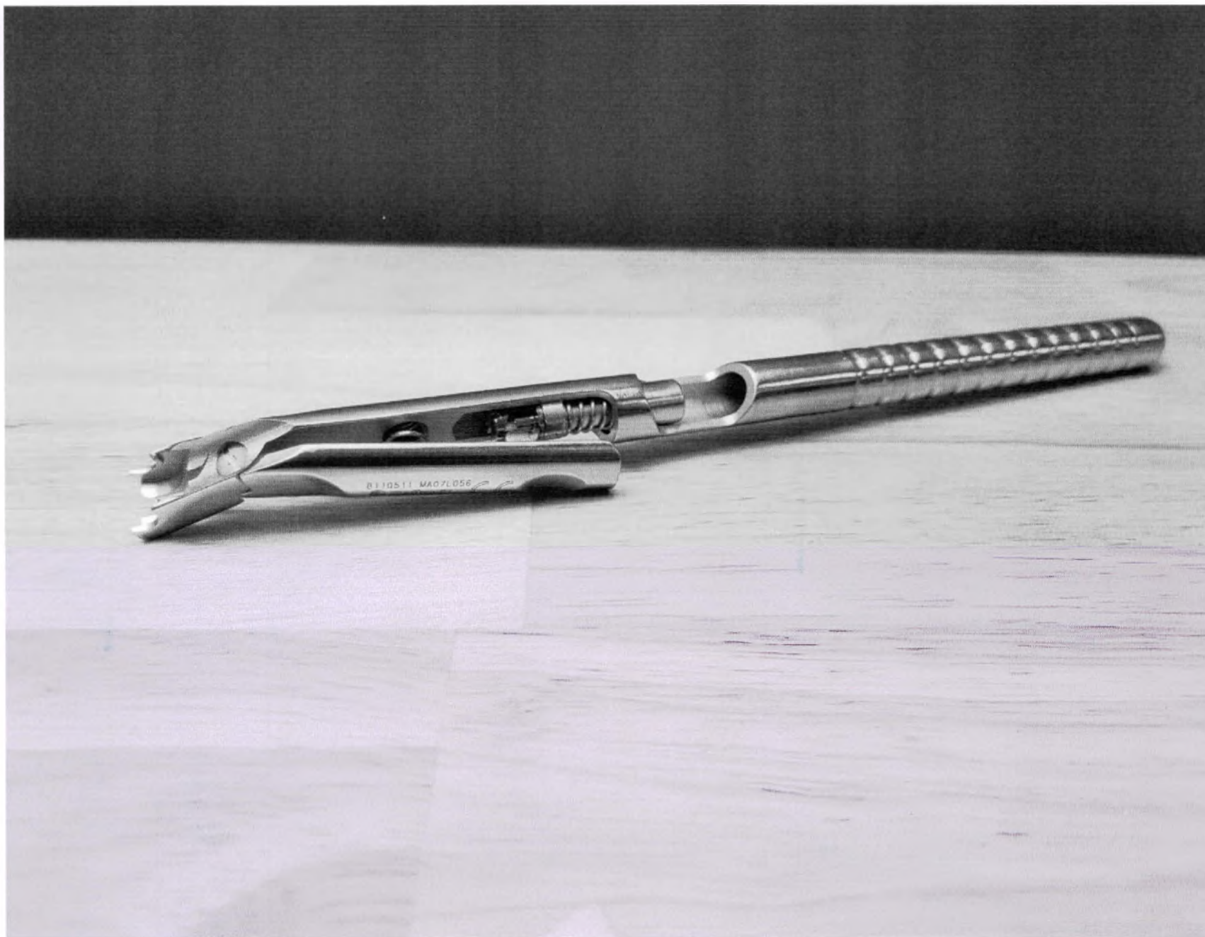
Держатель коннектора поперечного
