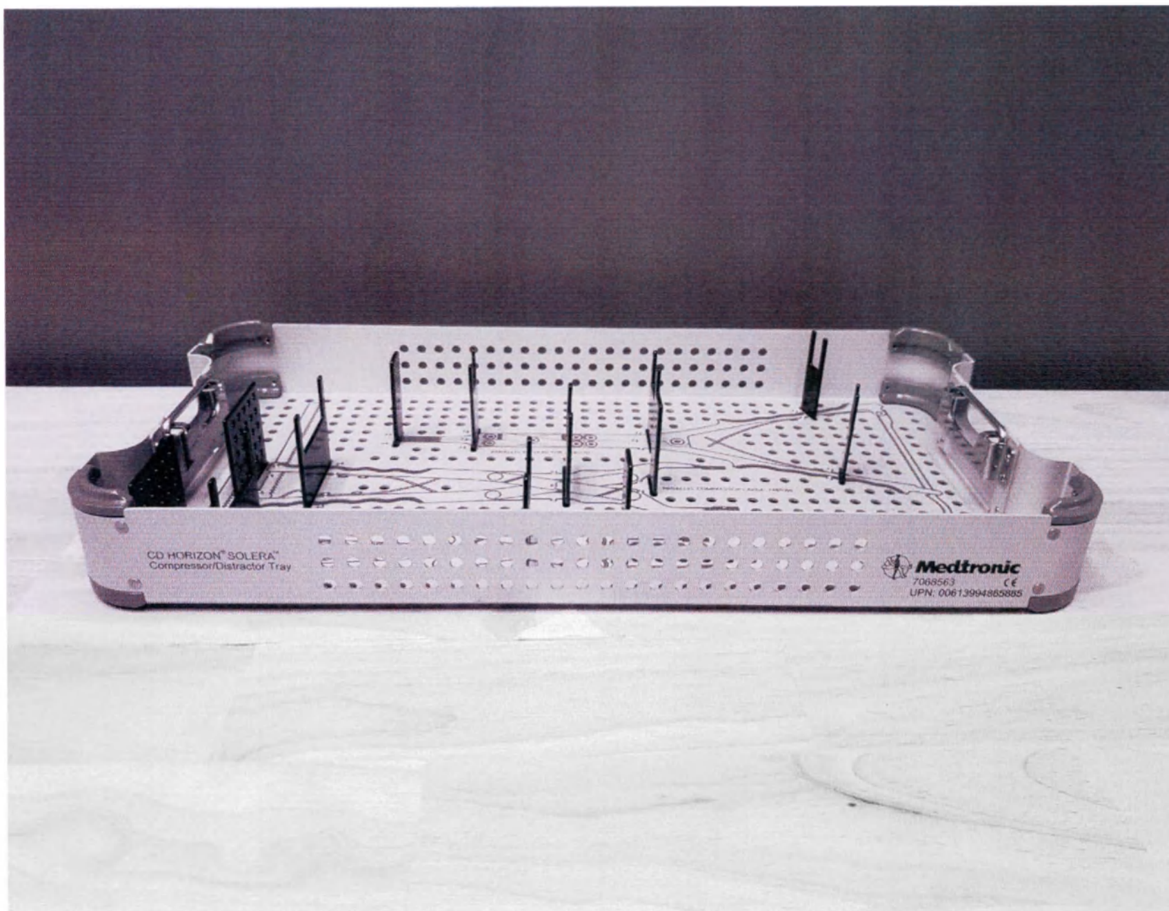
Полка для компрессоров и дистракторов
