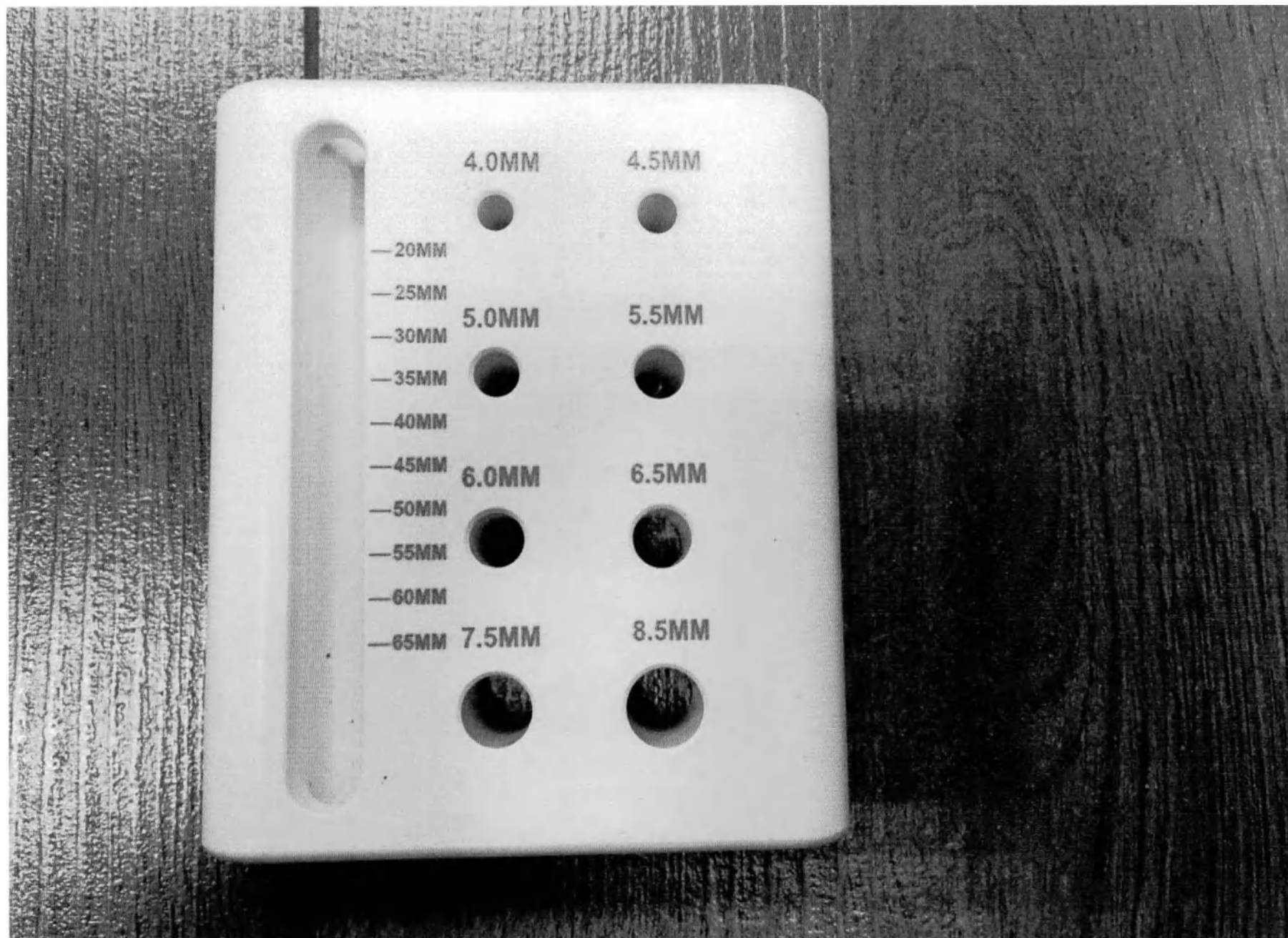
Шаблон полиаксиального транспедикулярного винта
