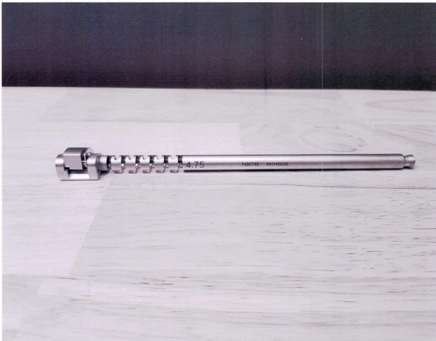
Гильза внешняя с замком 4,75 мм
