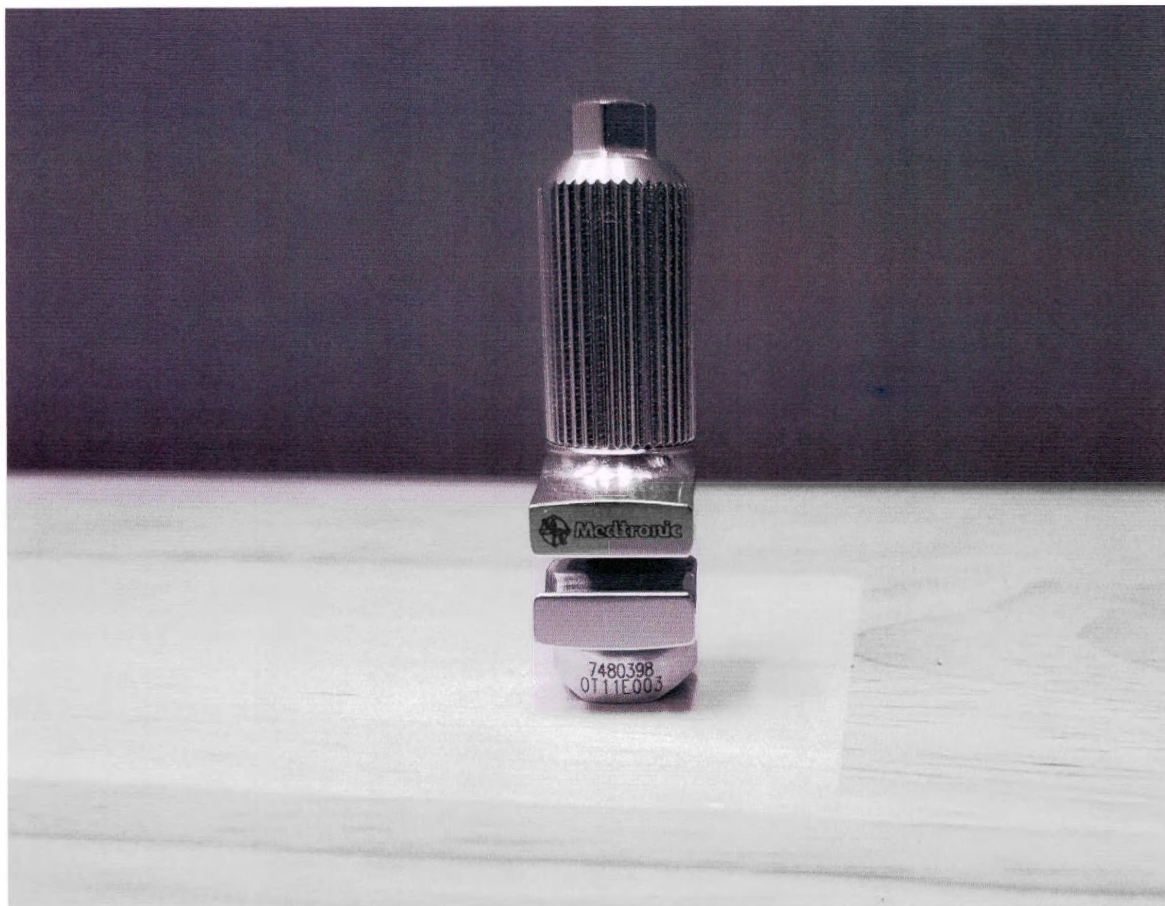
Муфта модуля деротационного
