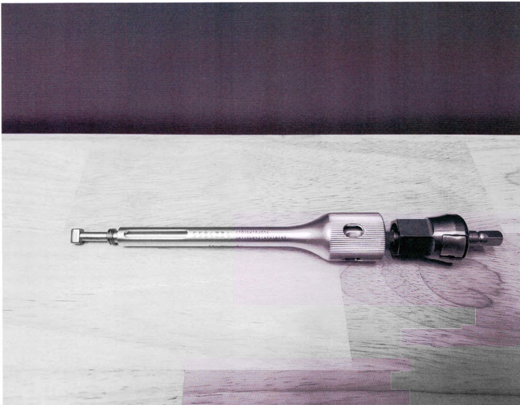
Вал отверточный с замком 5,5/6,0 мм
