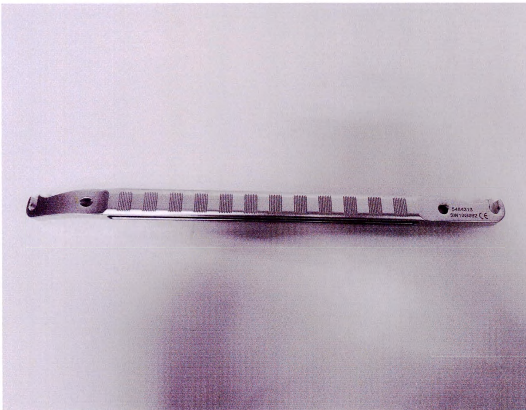
Сгибатель стержня "ин-ситу" (На примере варианта исполнения Сгибатель стержня "ин-ситу" левый 4,75 мм)
