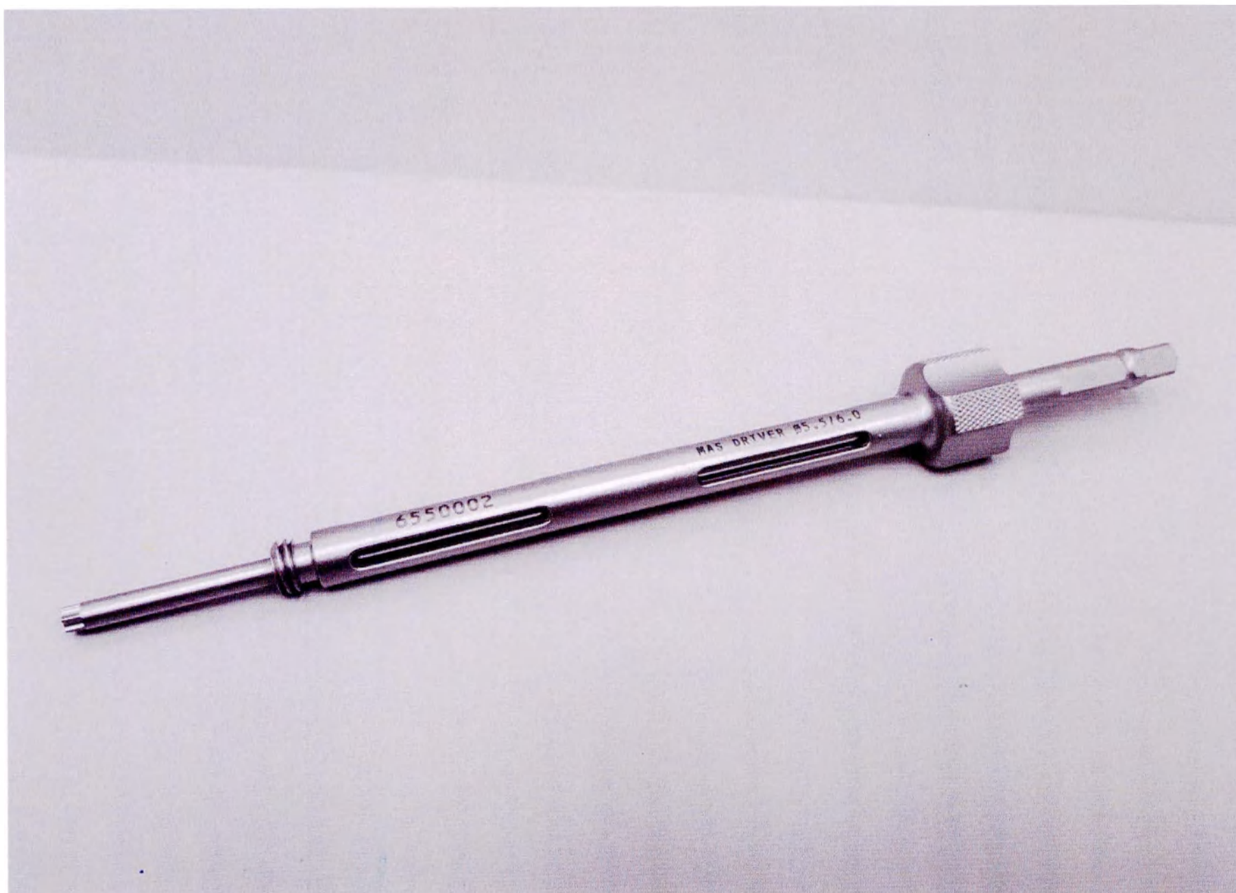
Вал отверточный удерживающий для полиаксиальных винтов 5,5/6,0 мм
