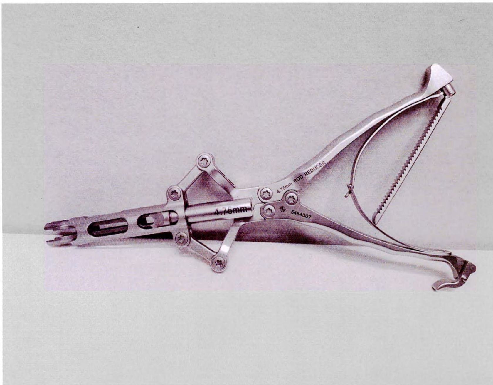
Редуктор Биля 4,75 мм
