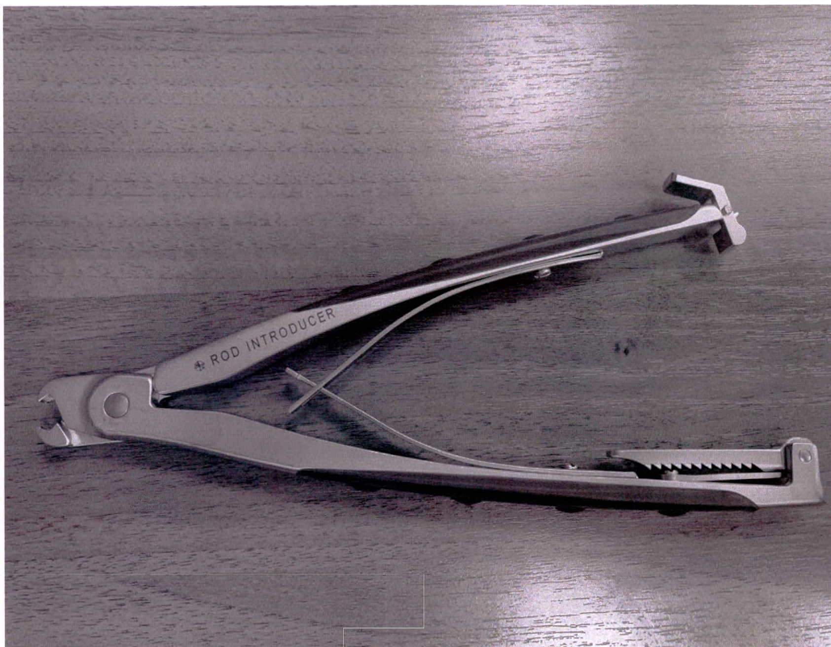
Инструмент для удерживания стержня 4,75 мм
