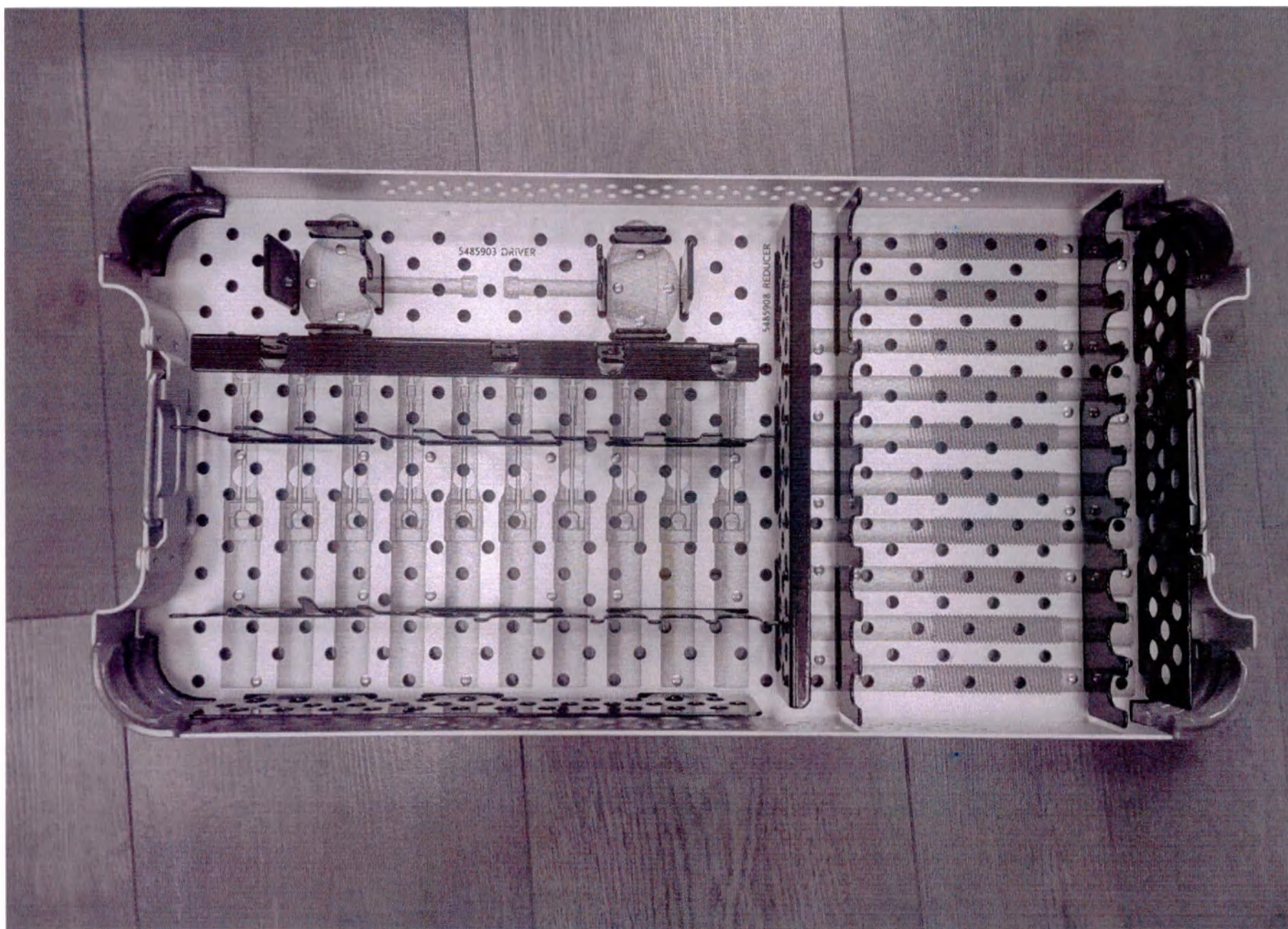
Полка EXTENDER SET
