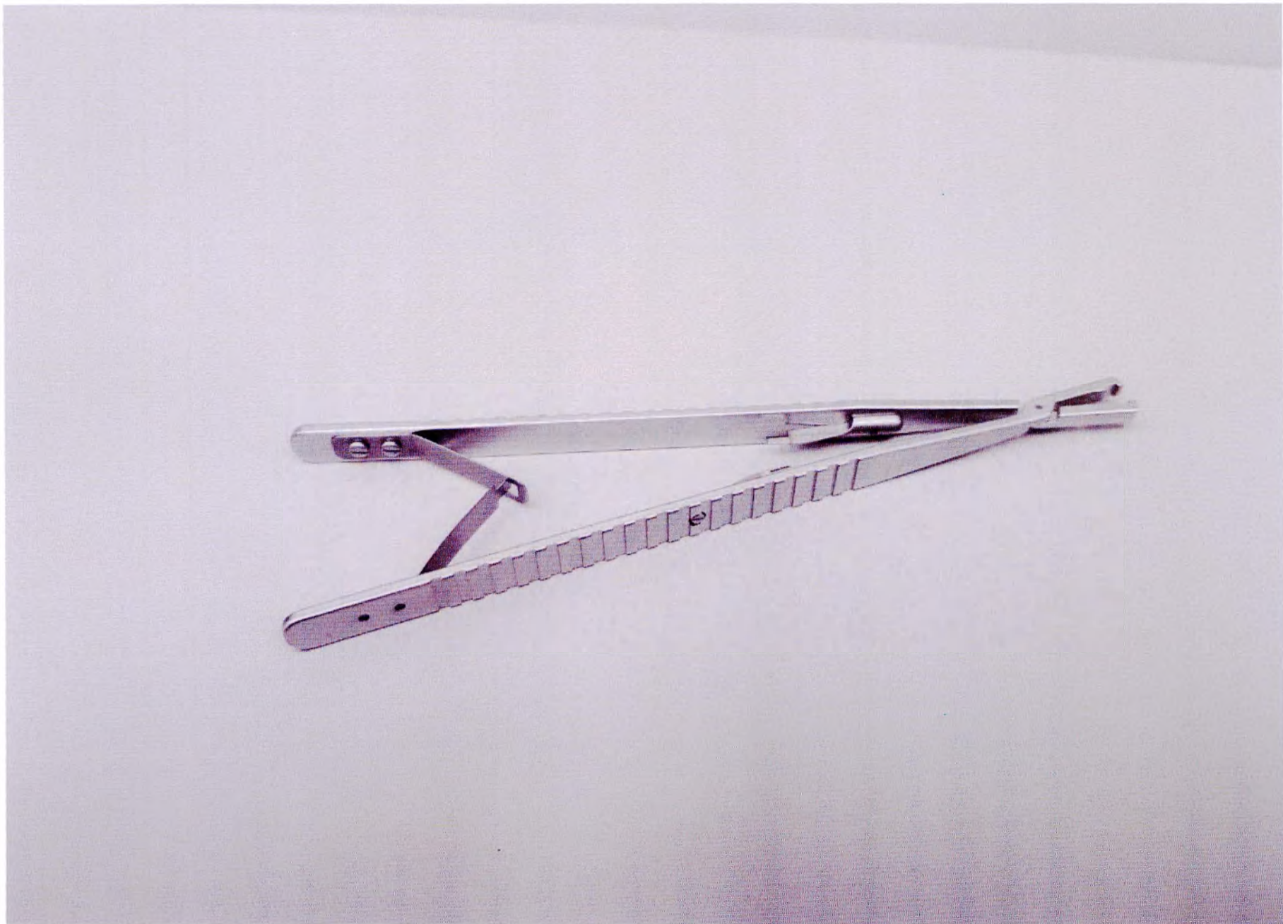
Держатель стержня шейный
