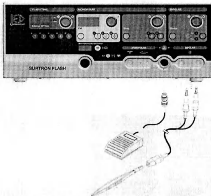
Типичная конфигурация для использования в биполярном режиме
