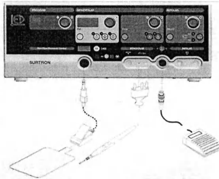
Типичная конфигурация для использования в монополярном режиме
