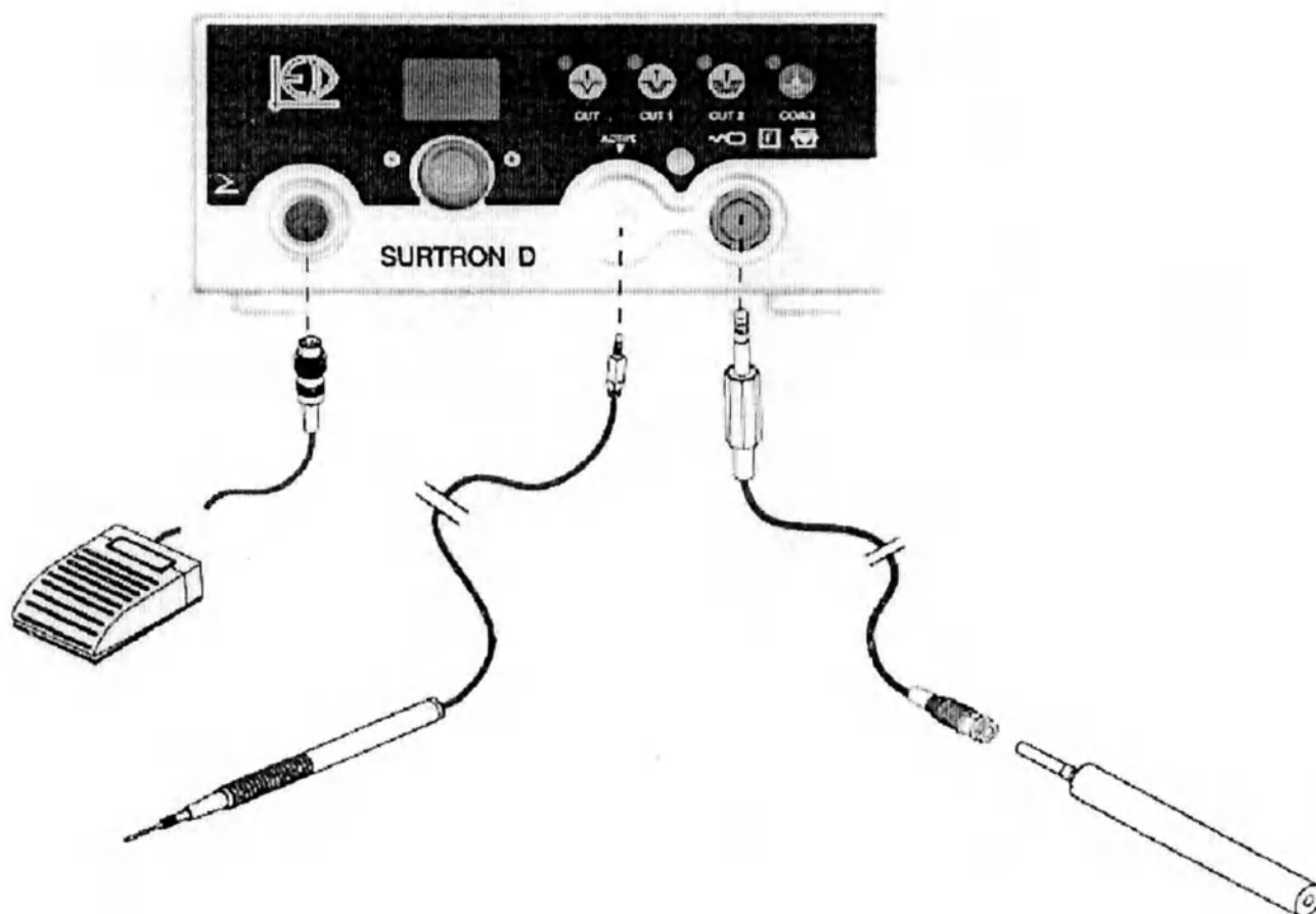
Типовая конфигурация Surtron 50 D
