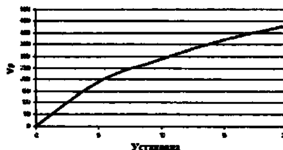
Диаграмма изменения максимального выходного напряжения MICRO в зависимости от V_p
