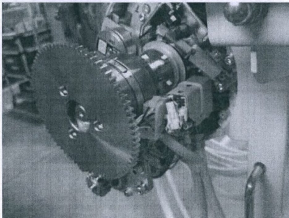
Блок автопозиционирования (до 4-х шт.)
