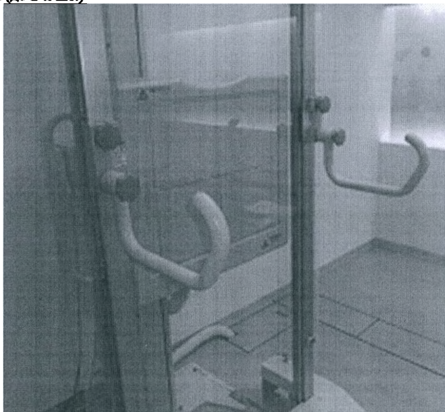
Вертикальная стойка с подножкой для пациента и боковыми захватами для рук для исследования в режиме автостичинга (до 2-х шт.)
