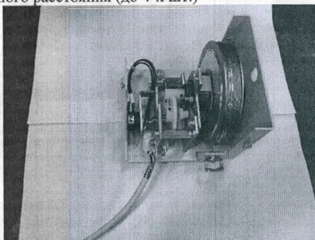
Продольный детектор фокусного расстояния (до 4-х шт.)
