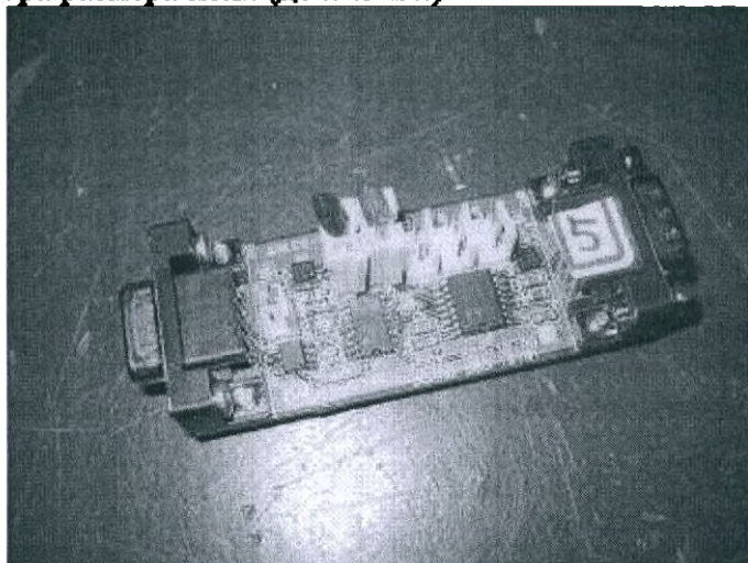
Блок автоматического выбора размера поля (до 2-х шт.)
