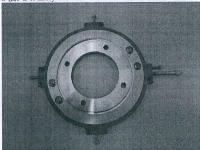
Блок поворота коллиматора (до 2-х шт.)
