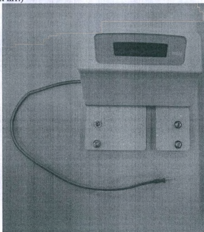
Монтажный комплект дозиметра (до 2-х шт.)
