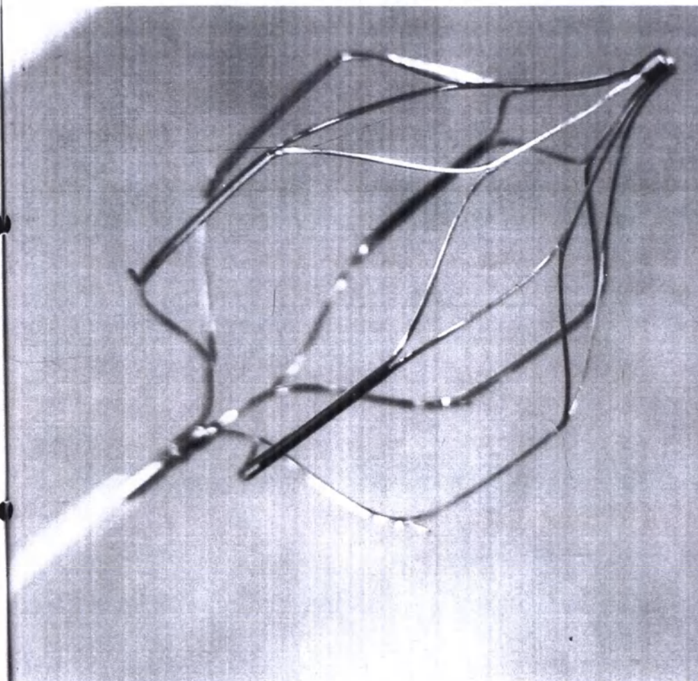
Кава-фильтр венозный Aegisy с системой доставки. Внешний вид фильтра.
