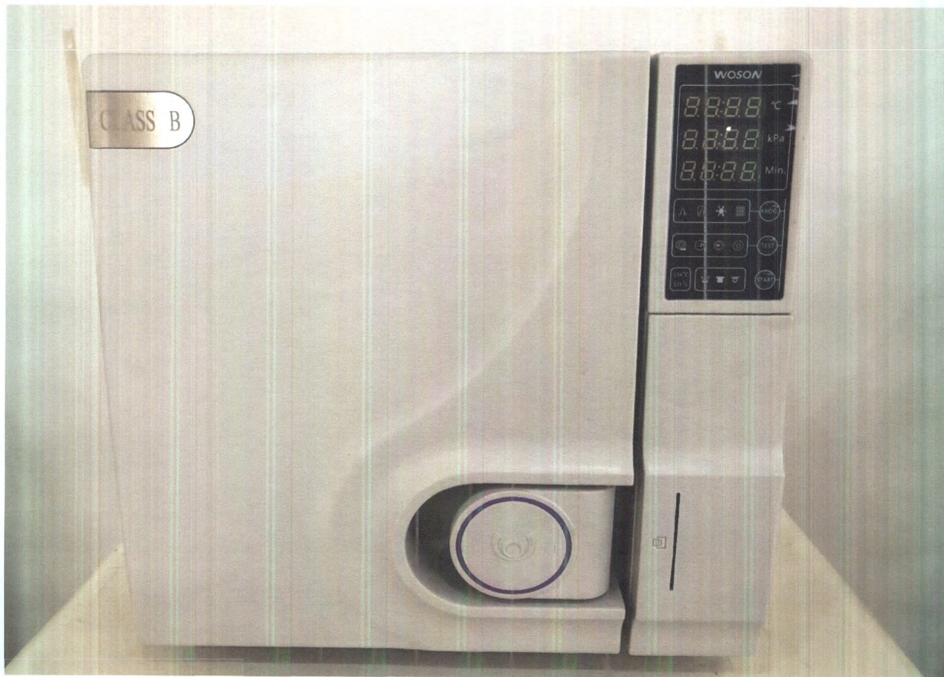
Стерилизатор стоматологический паровой Восон (Woson), вариант исполнения Танко 12Л (Tanco 12L)
