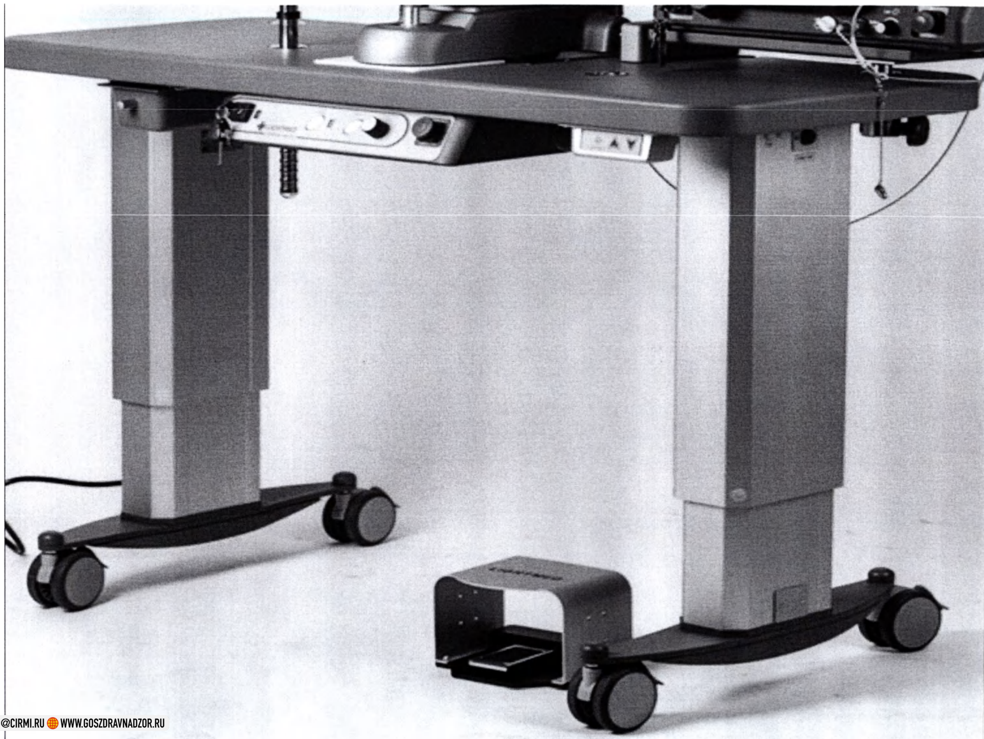
29. Моторизованный стол с крышкой с боковыми подъемными колоннами.
