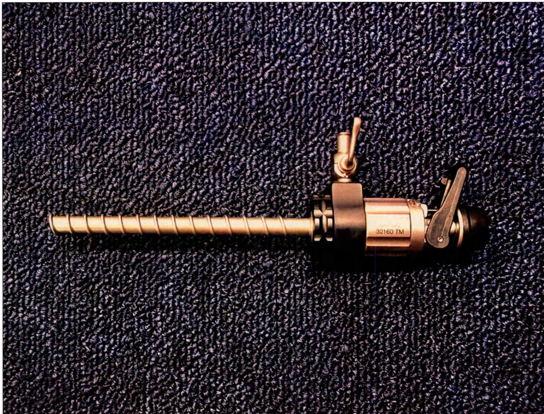
Рис. 109. Троакар в собранном виде на примере варианта исполнения 30160TMR: Троакар TERNAMIAN EndoTIP, с multifunctional клапаном, диаметр 6 мм, длина 10,5 см. Имеет схожий внешний вид, отличается цветовой маркировкой с каталожными номерами изделий вариантов исполнения: 30160TKR, 30160TMR, 30103TMR, 30117MT
