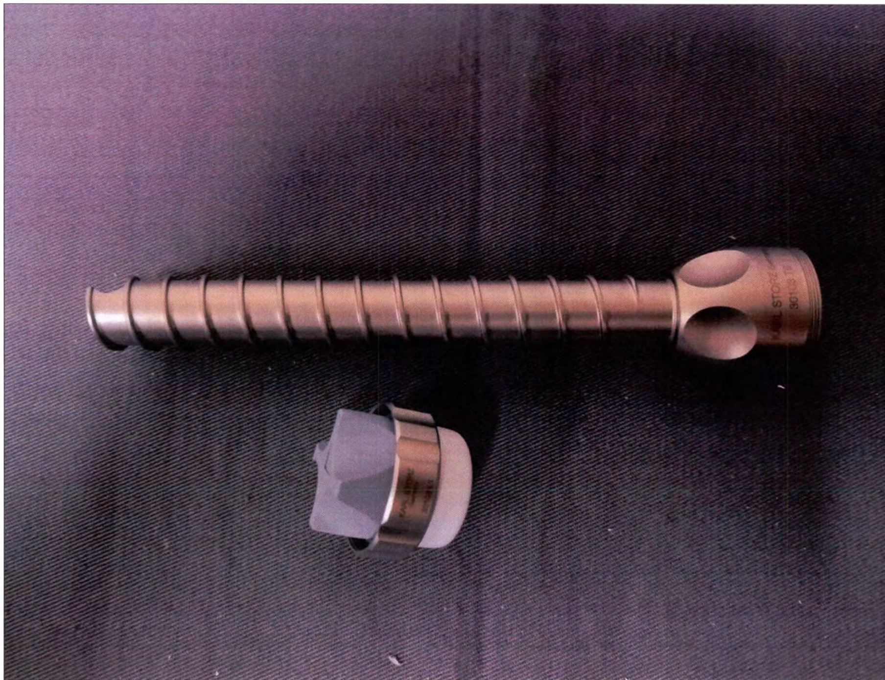
Рис. 117. Троакар в разобранном виде на примере варианта исполнения 30103ML : Троакар TERNAMIAN EndoTIP, с лепестковым клапаном, диаметр 11 мм, длина 10,5 см.
