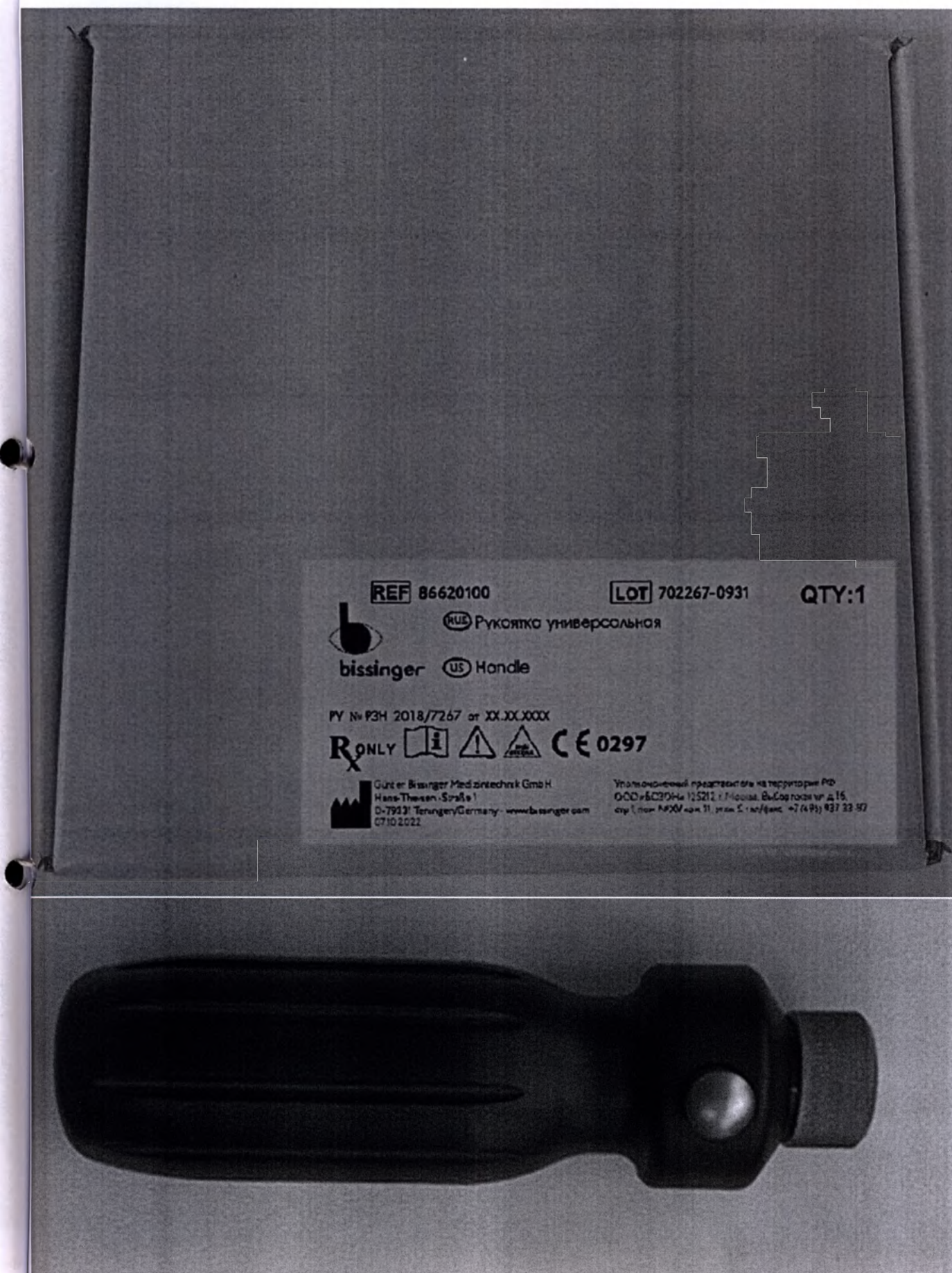
Фото 9. Рукоятка универсальная, 86620100.
