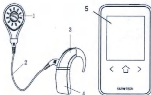
1 Передающая катушка; 2 Передающий кабель; 3 Блок обработки сигналов; 4 Отсек аккумуляторный батарейный для заушного типа ношения; 5 Пульт дистанционного управления
