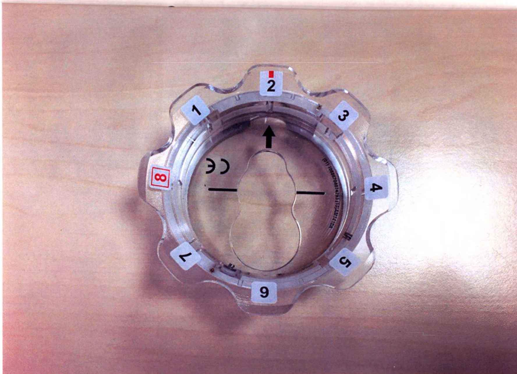
Локатор. Часть программатора CODMAN CERTAS
