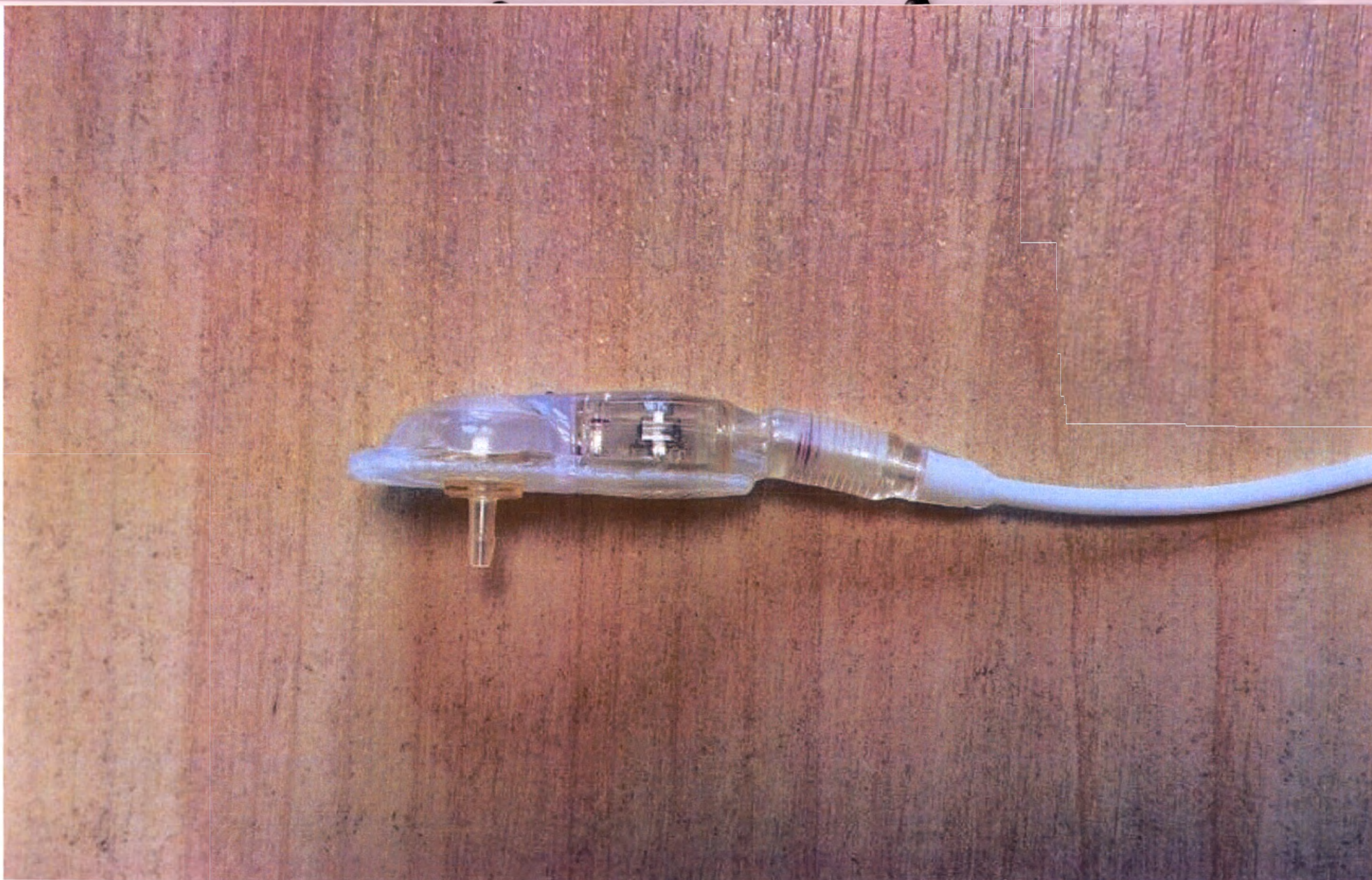
Внешний боковой вид клапана под трепанационное отверстие, входящего в состав варианта исполнения 23
