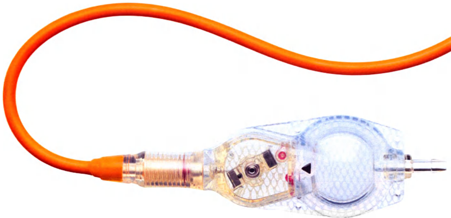
Внешний вид клапана со встроенным дистальным катетером BACTISEAL, входящего в состав варианта исполнения 6
