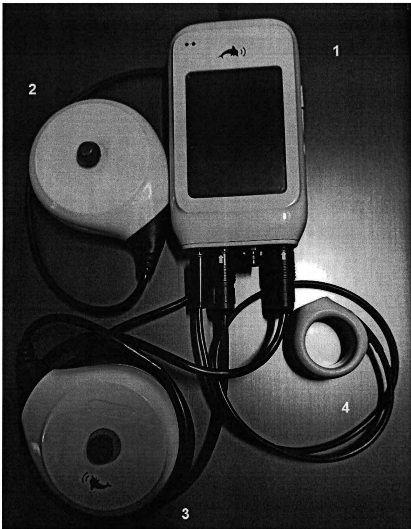
Рисунок 2– «Монитор фетальный портативный «Илифия», вариант исполнения «Илифия-Д» по ТУ 26.60.12-001-30176328-2020»
