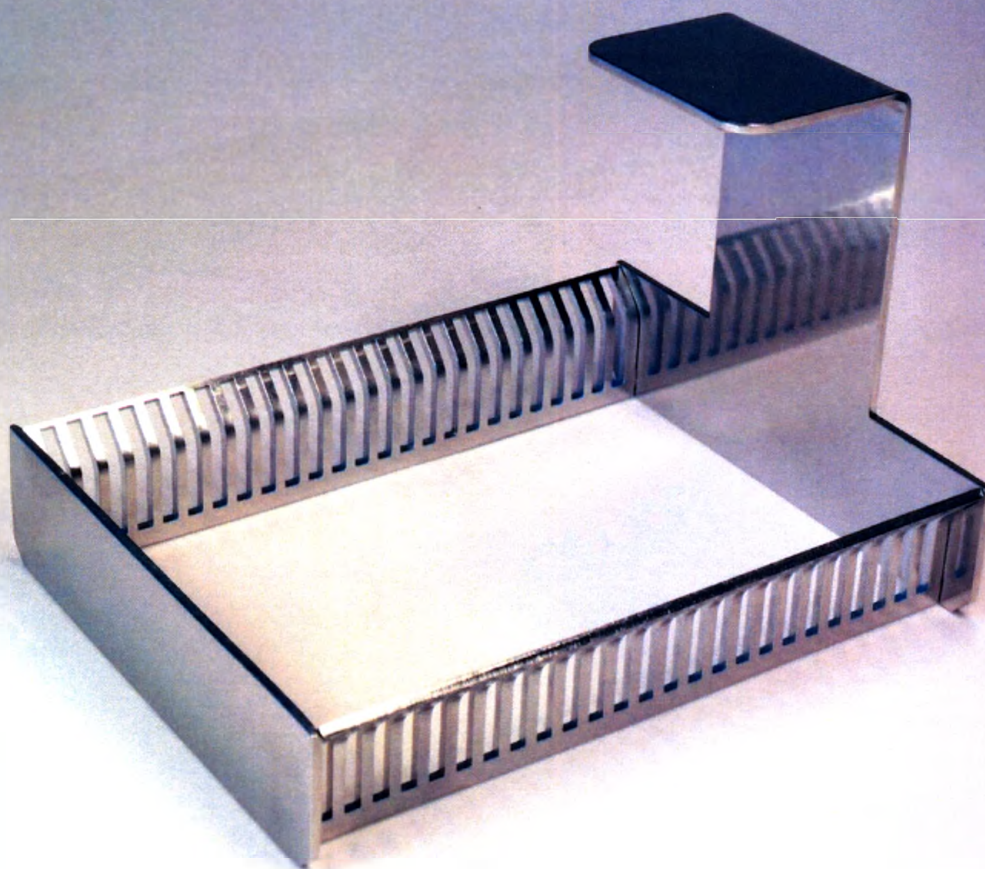
Штатив для предметных стекол универсальный ШУ-25 (02.23.00)
