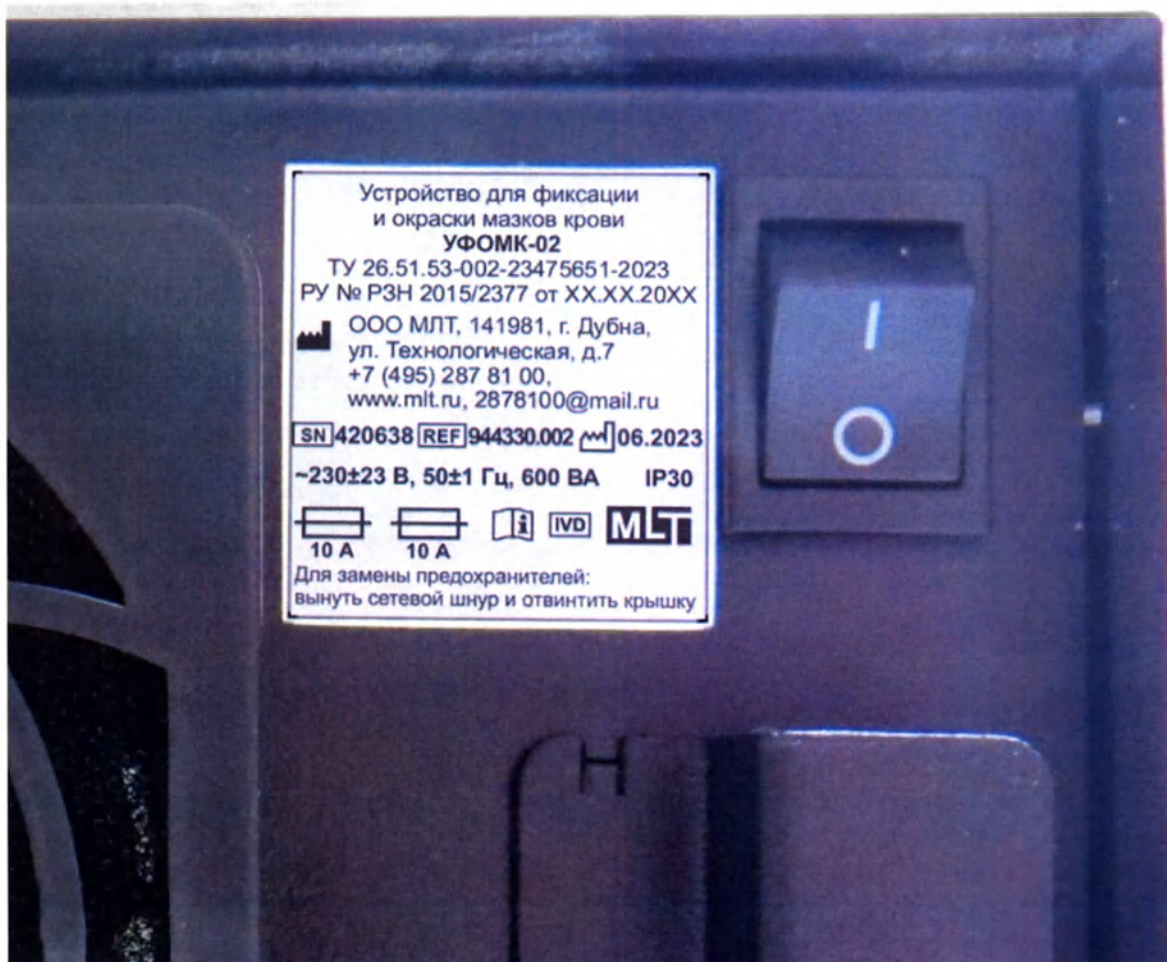
Устройство для фиксации и окраски мазков крови УФОМК-02 (заводская табличка)
