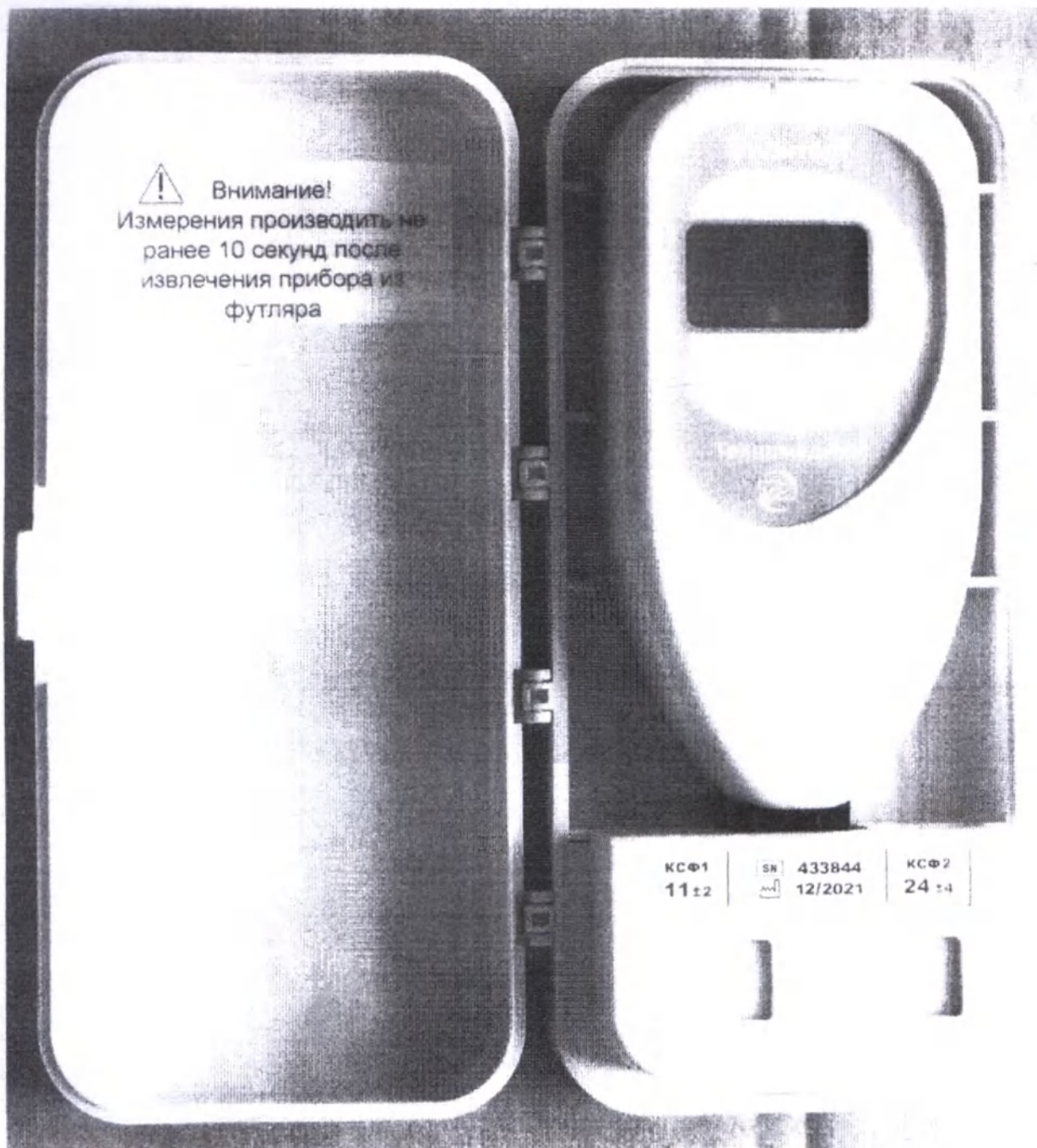
Прибор в футляре со встроенными контрольными светофильтрами КСФ1 и КСФ2
