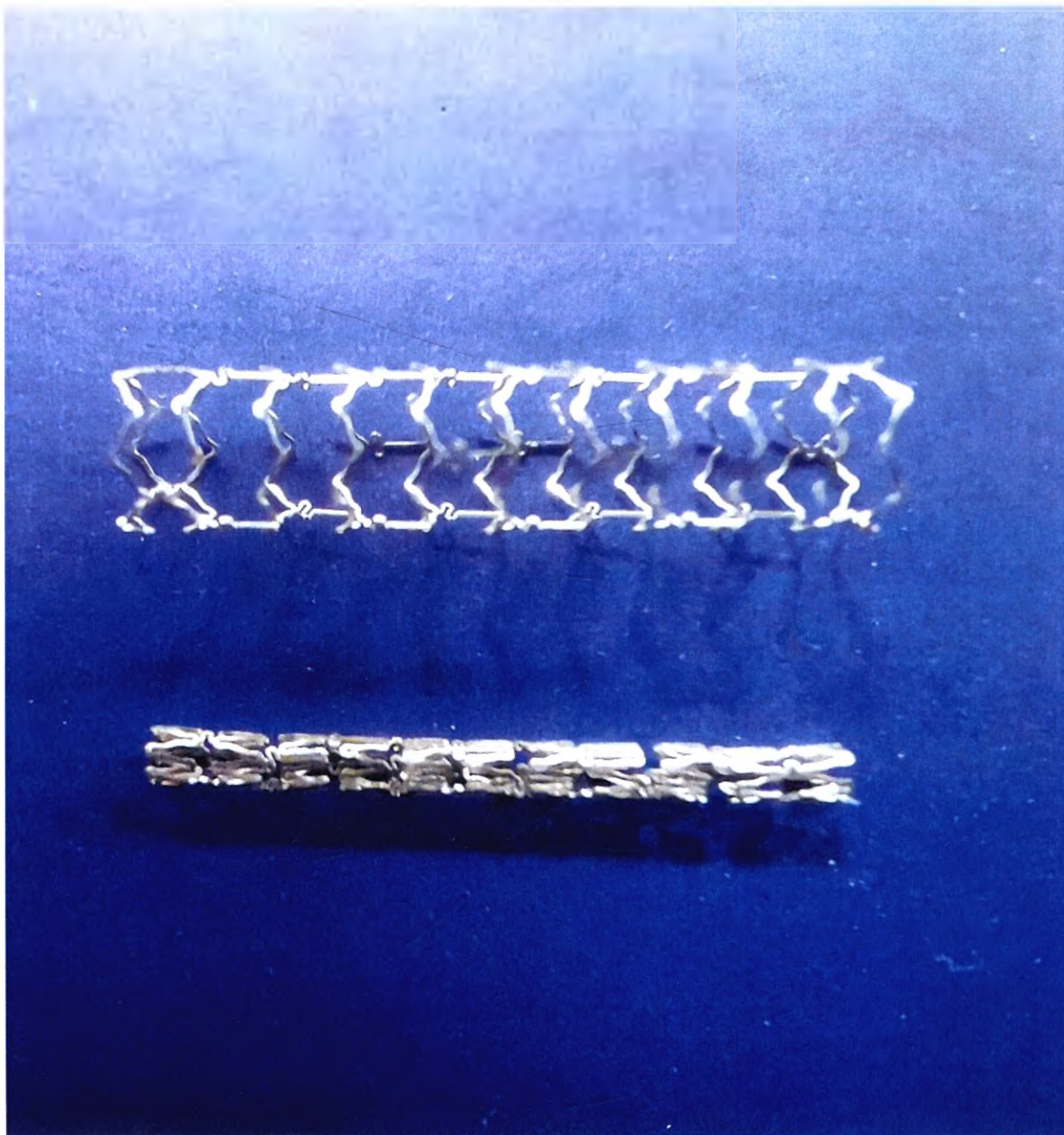
1. Общий вид изделия «Система кобальт-хромового коронарного стента Firebird2™ с лекарственным покрытием (рапамицин)» до расширения (вид снизу) и после расширения баллоном (вид сверху).
