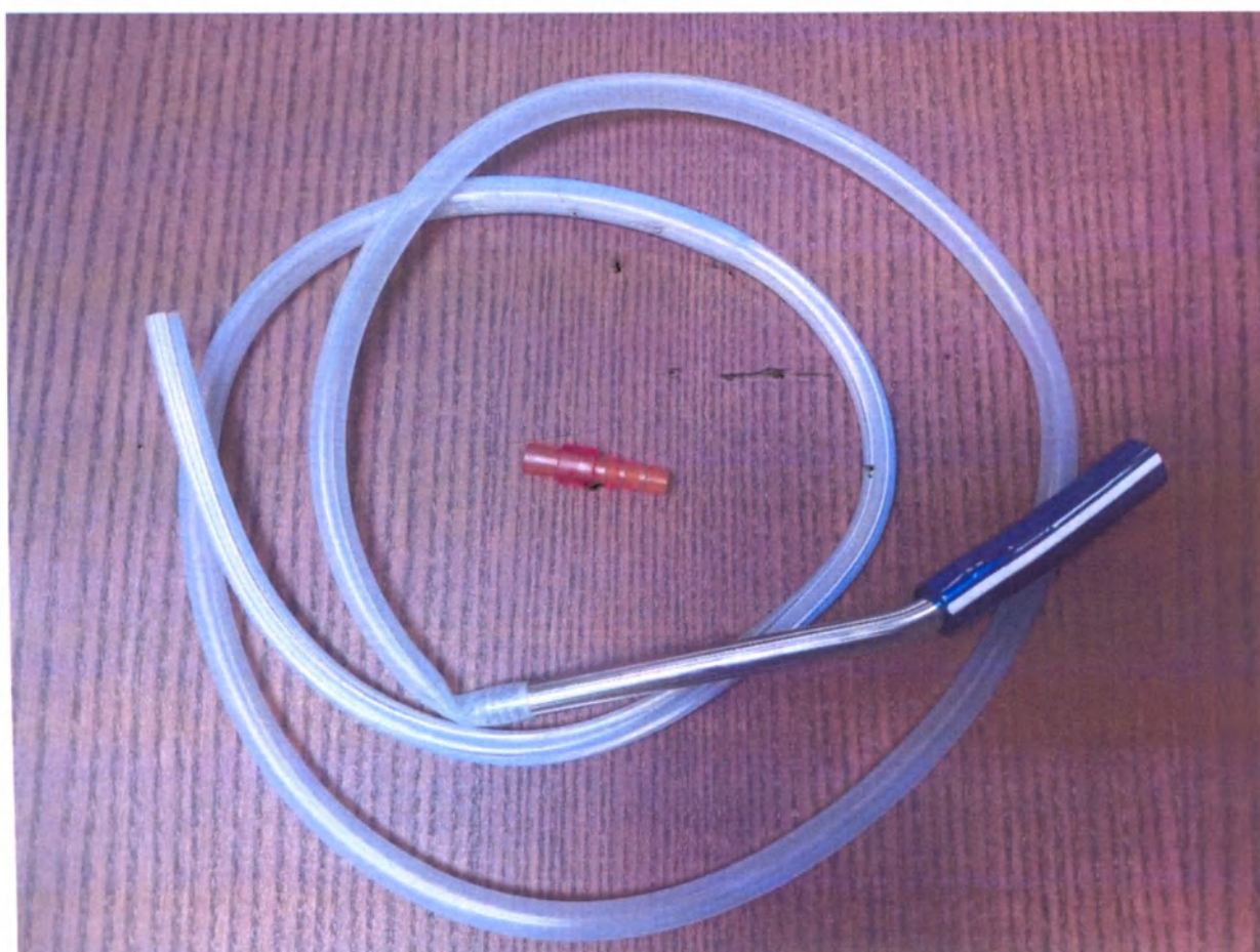
Рисунок 15 Трубка дренажная силиконовая, круглая с пазами, со стилетом, с коннектором L, длина 1200 мм, размер CH/FR: 24
