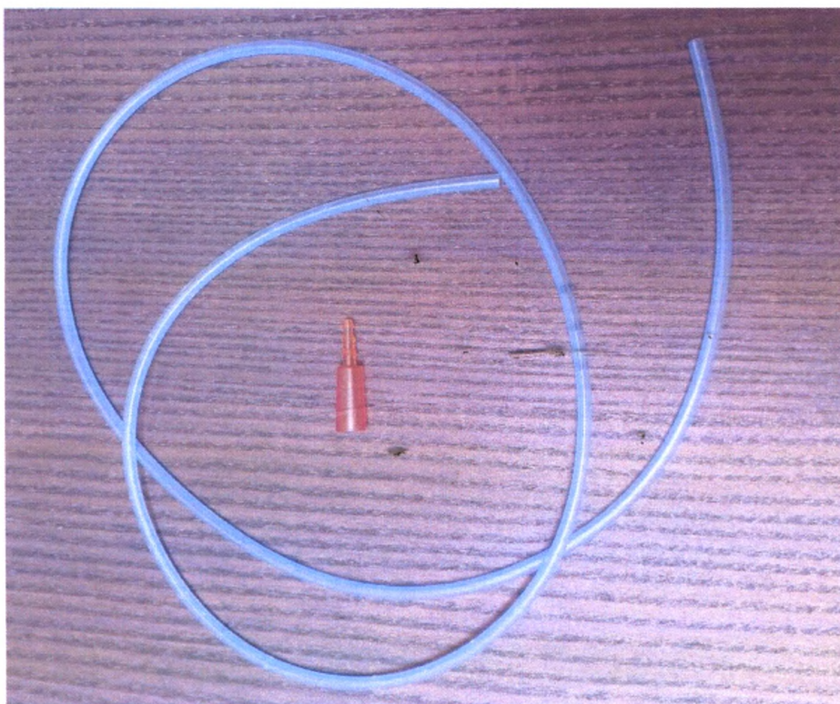
Рисунок 7 Трубка дренажная силиконовая, круглая с перфорацией, с коннектором XS, длина 900 мм, размер CH/FR: 10
