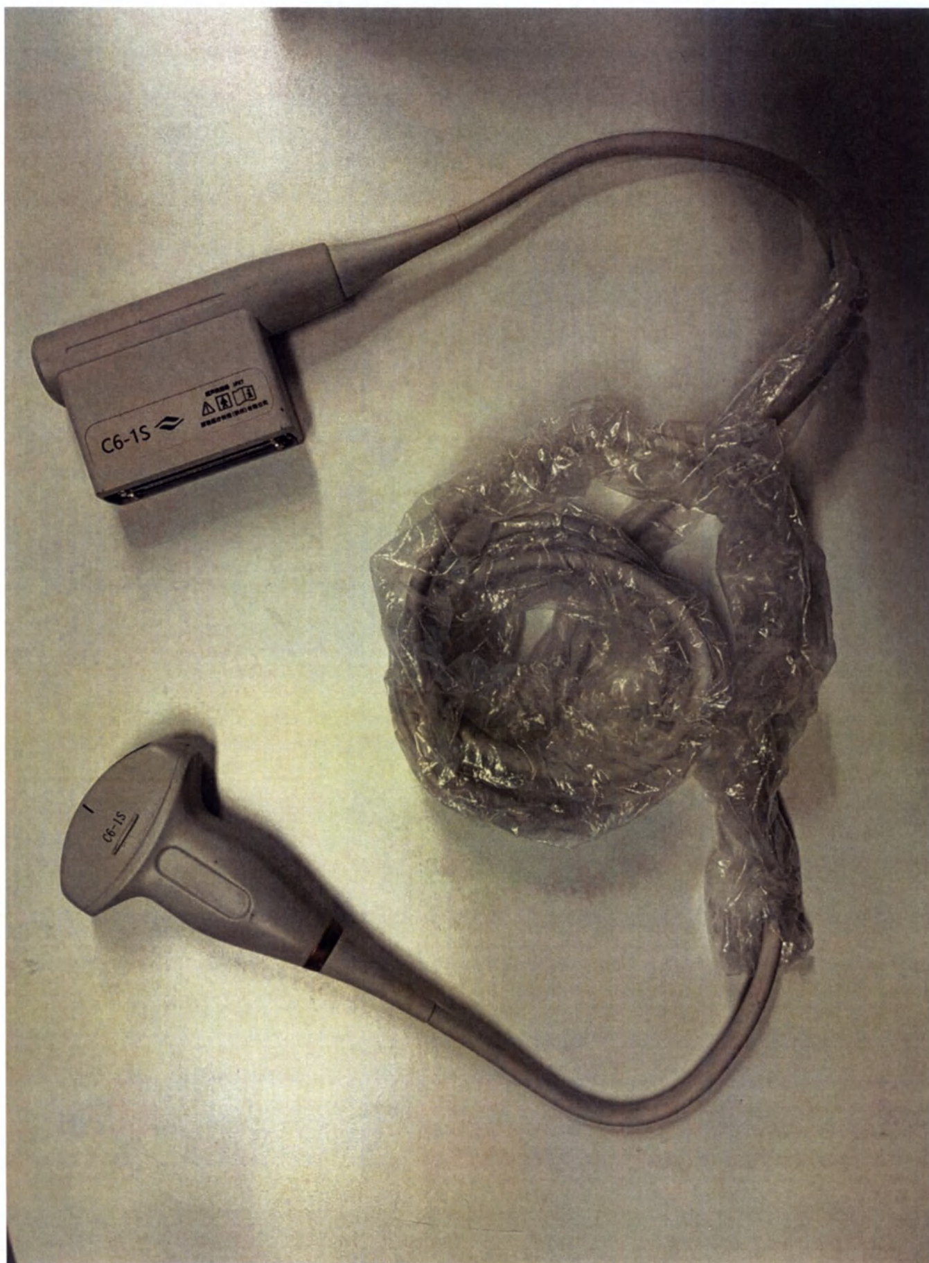
Рисунок 5 – Датчик конвексный C6-1S
