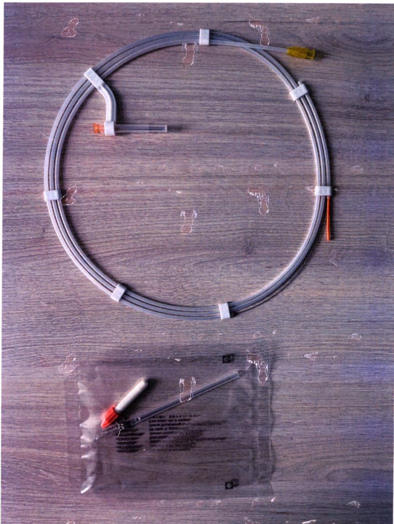
Содержание индивидуальной упаковки Проводника с гидрофильным покрытием Traxcess 14EX (проводник в защитном ободе, формирующий мандрен, инструмент для введения проводника и устройство закручивающее)
