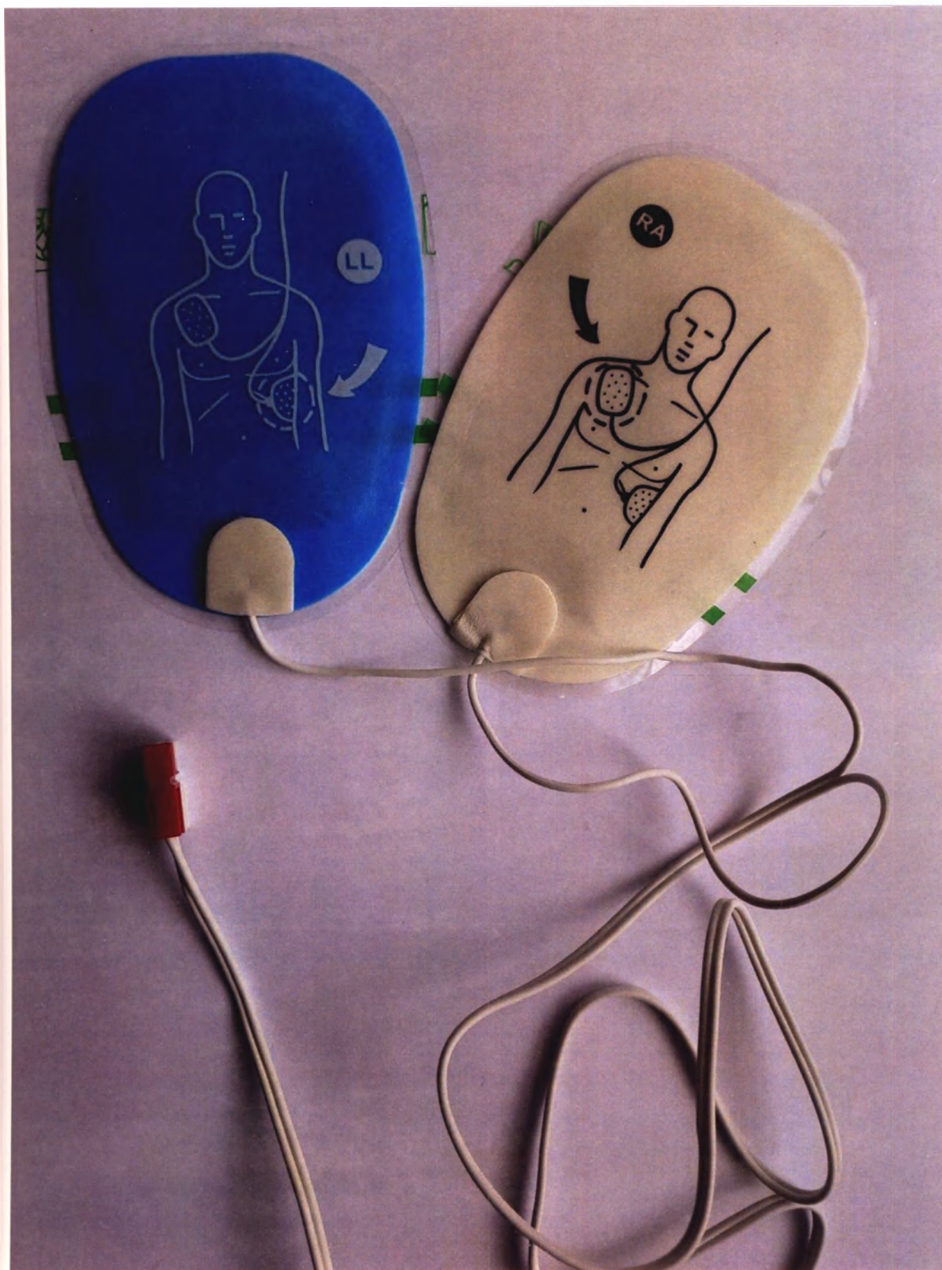
Рисунок 8 — Электрод дефибрилляции OBS-DE/P, артикул 303A1525
