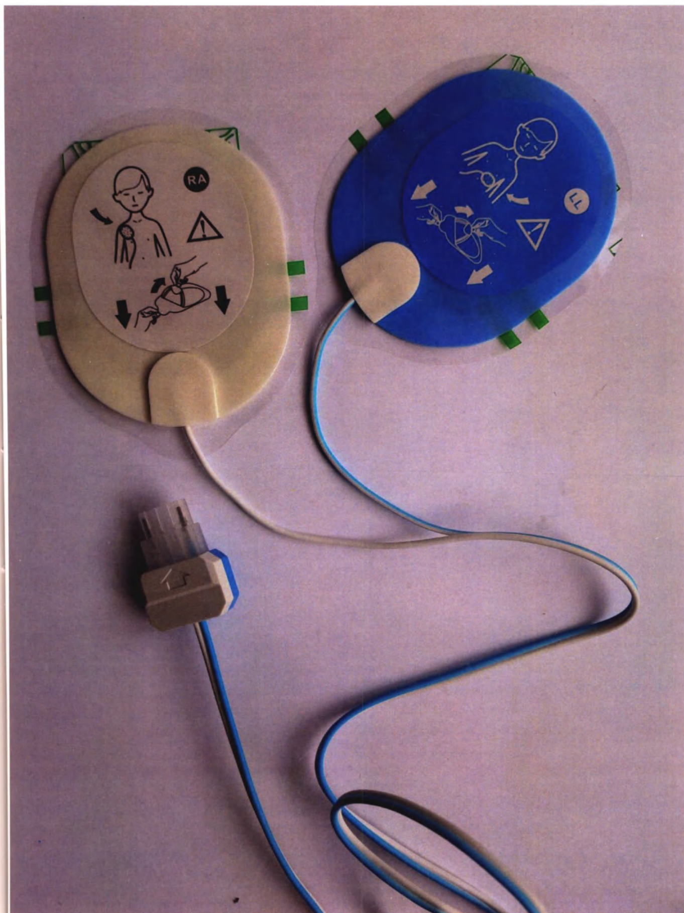
Рисунок 17 — Электрод дефибрилляции OBS-DE/W, артикул 303A4530
