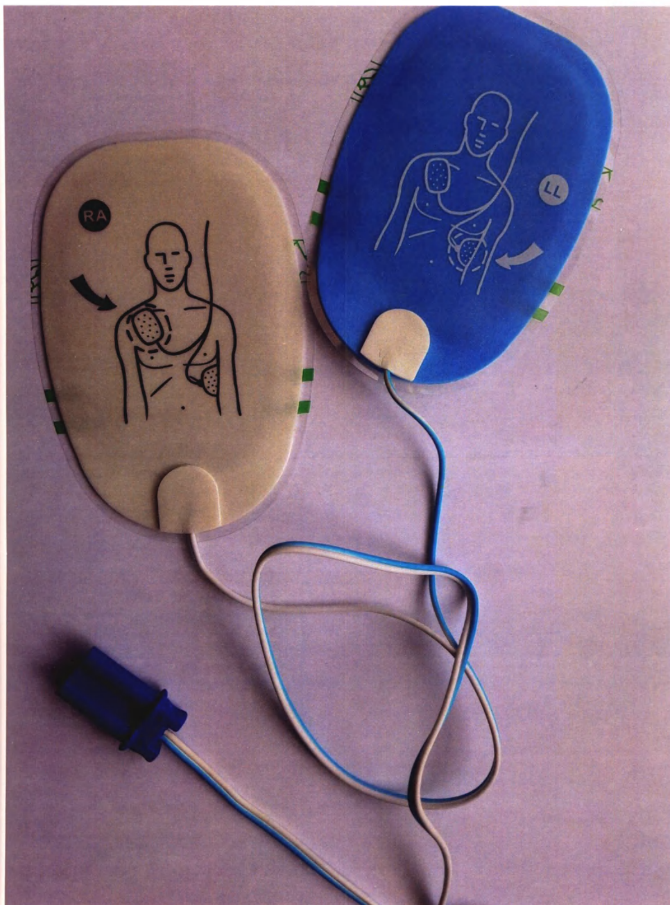
Рисунок 12 — Электрод дефибрилляции OBS-DE/P, артикул 303A4525
