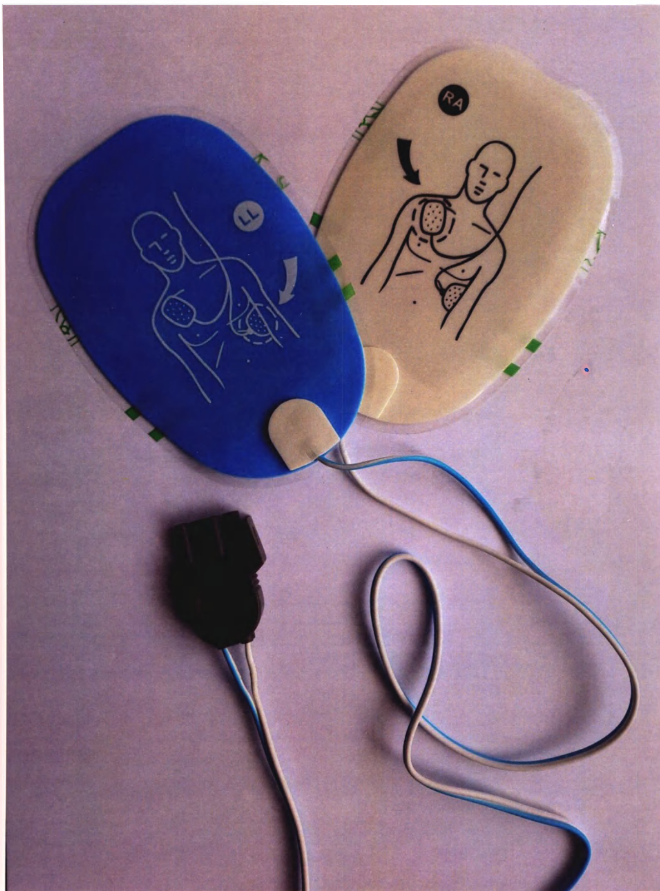
Рисунок 4 — Электрод дефибрилляции OBS-DE/P, артикул 303A5035
