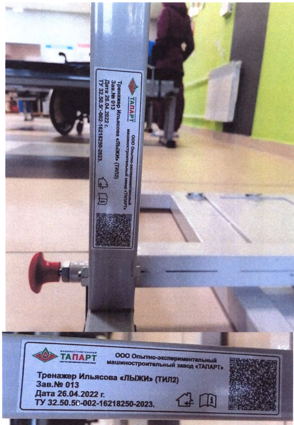
Фотографическое изображение 3 – Маркировка изделия . Тренажер Ильясова «ЛЫЖИ» (ТИЛ2)
